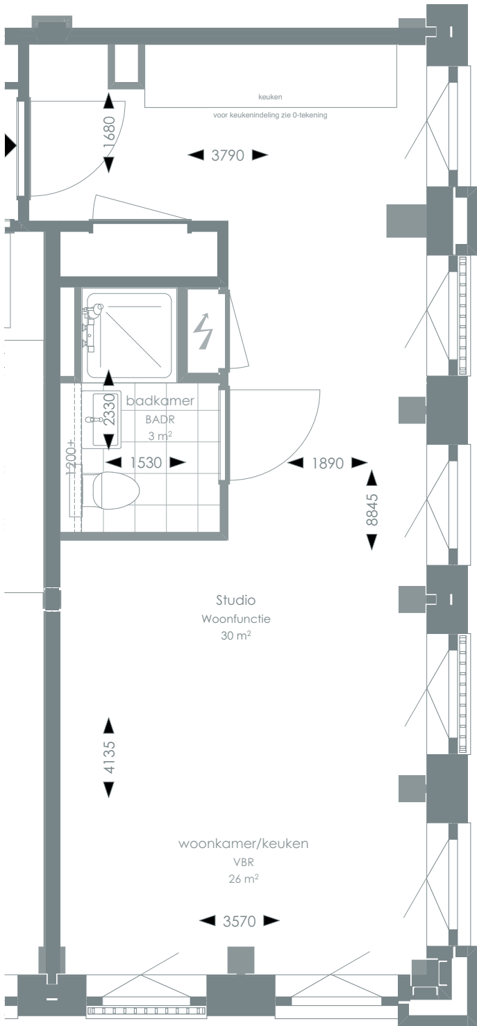
1:50 PLATTEGROND
