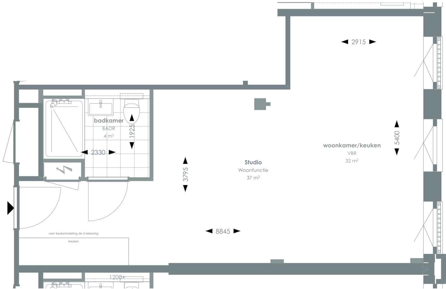
1:50 PLATTEGROND
