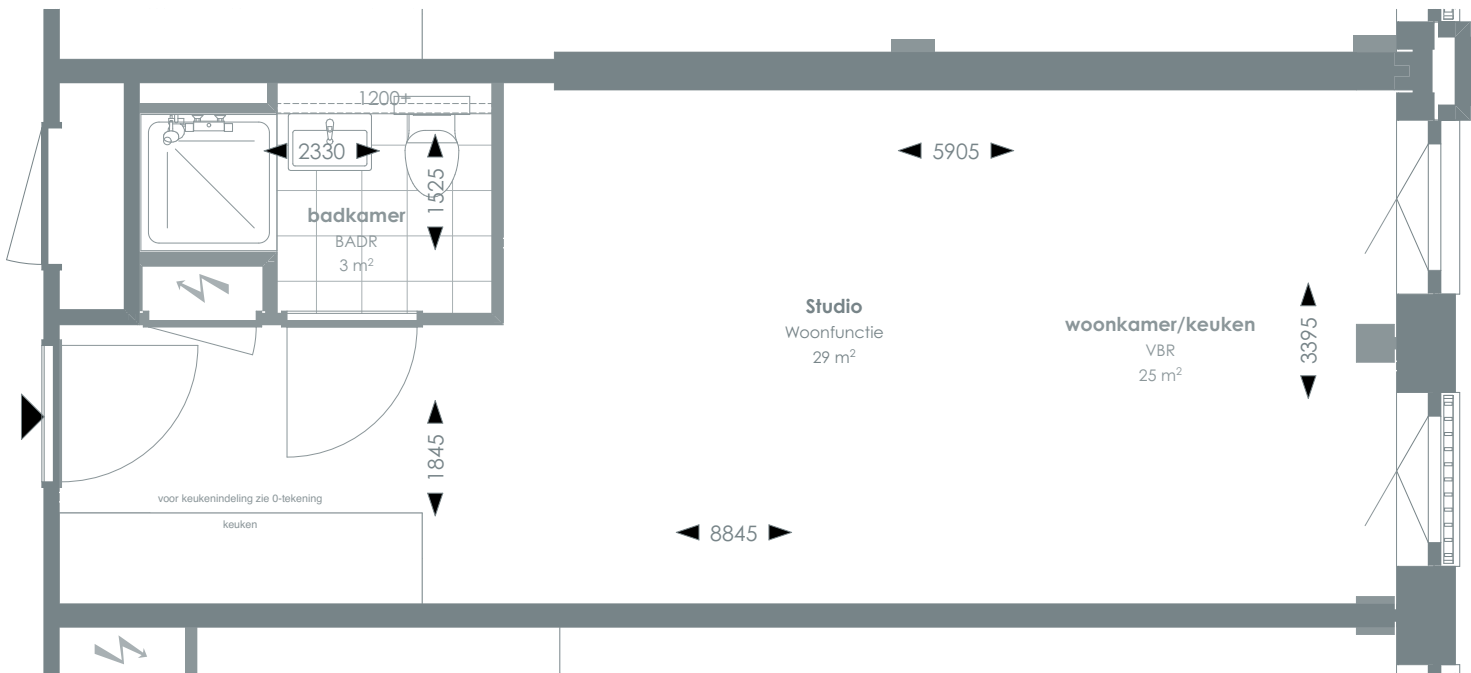
1:50 PLATTEGROND
