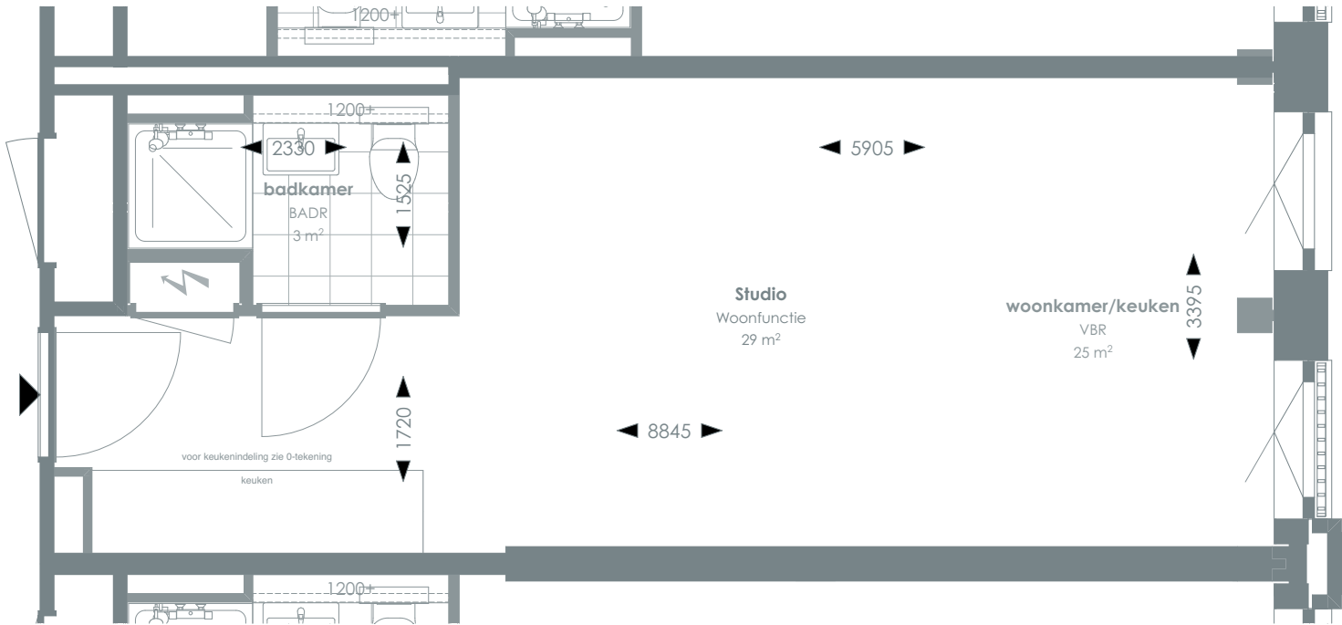
1:50 PLATTEGROND
