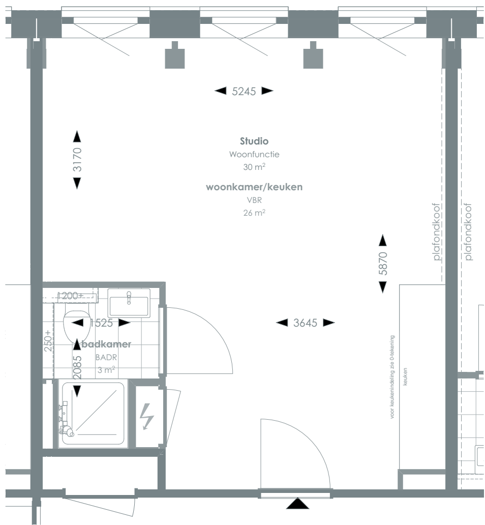
1:50 PLATTEGROND
