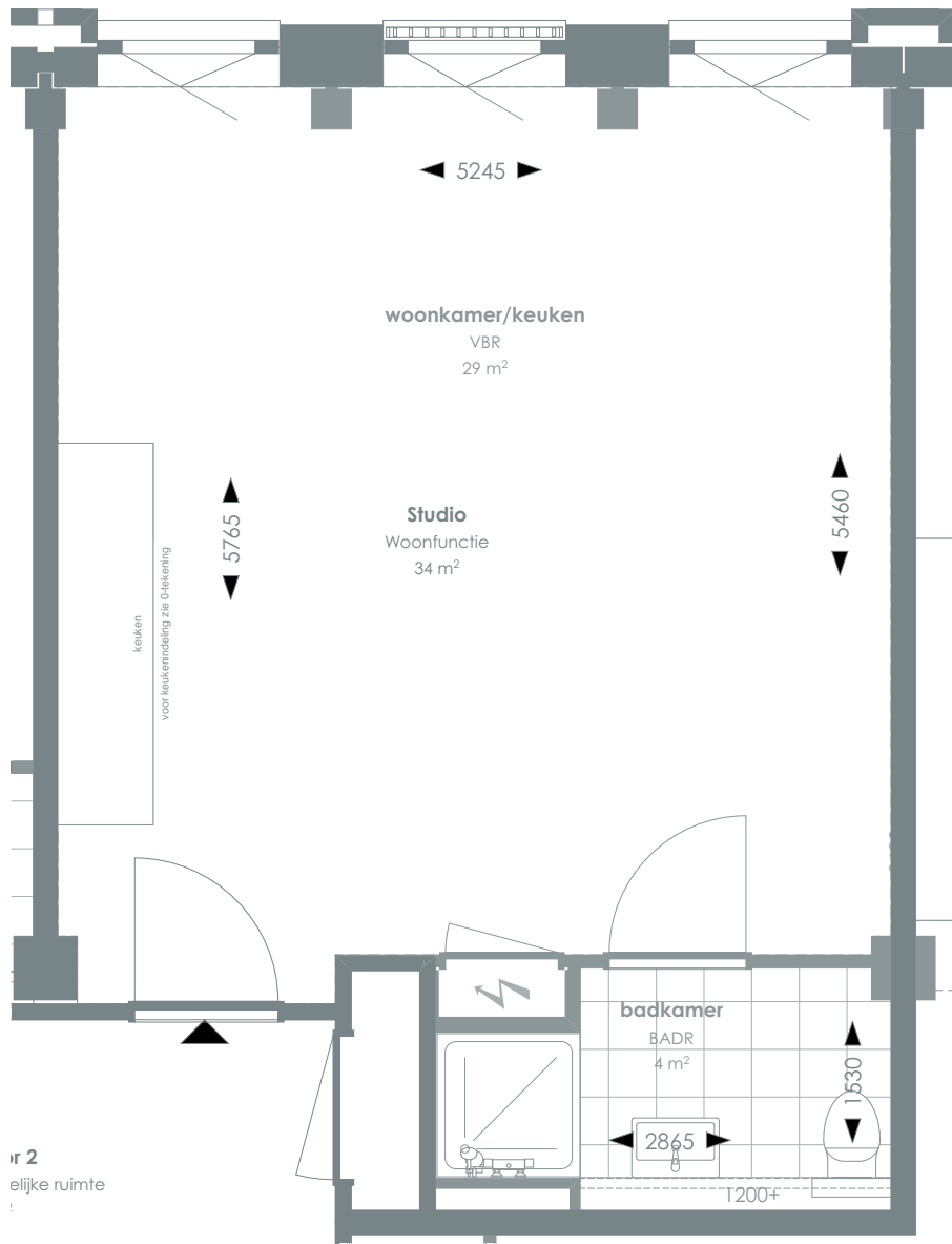
1:50 PLATTEGROND
