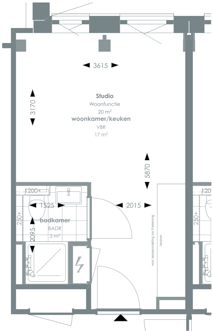
1:50 PLATTEGROND
