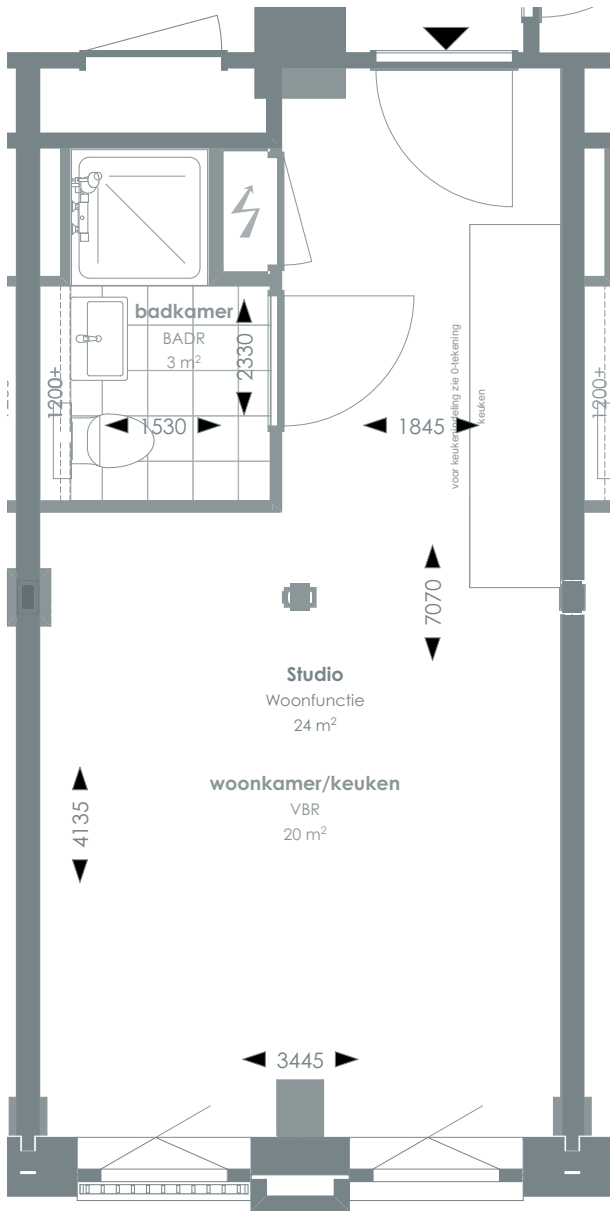
1:50 PLATTEGROND
