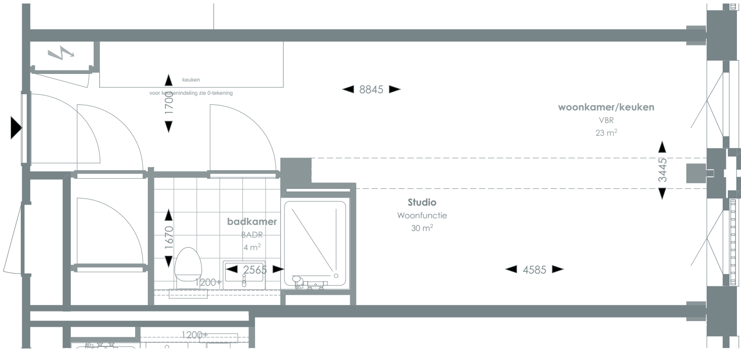
1:50 PLATTEGROND
