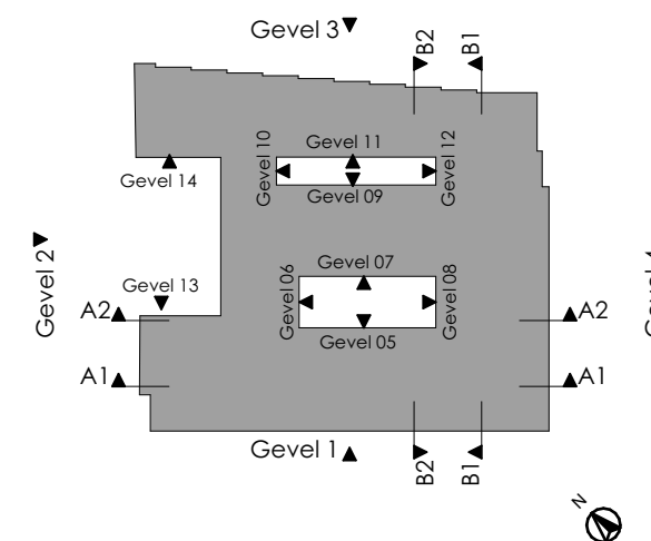
GEBOUWOVERZICHT
