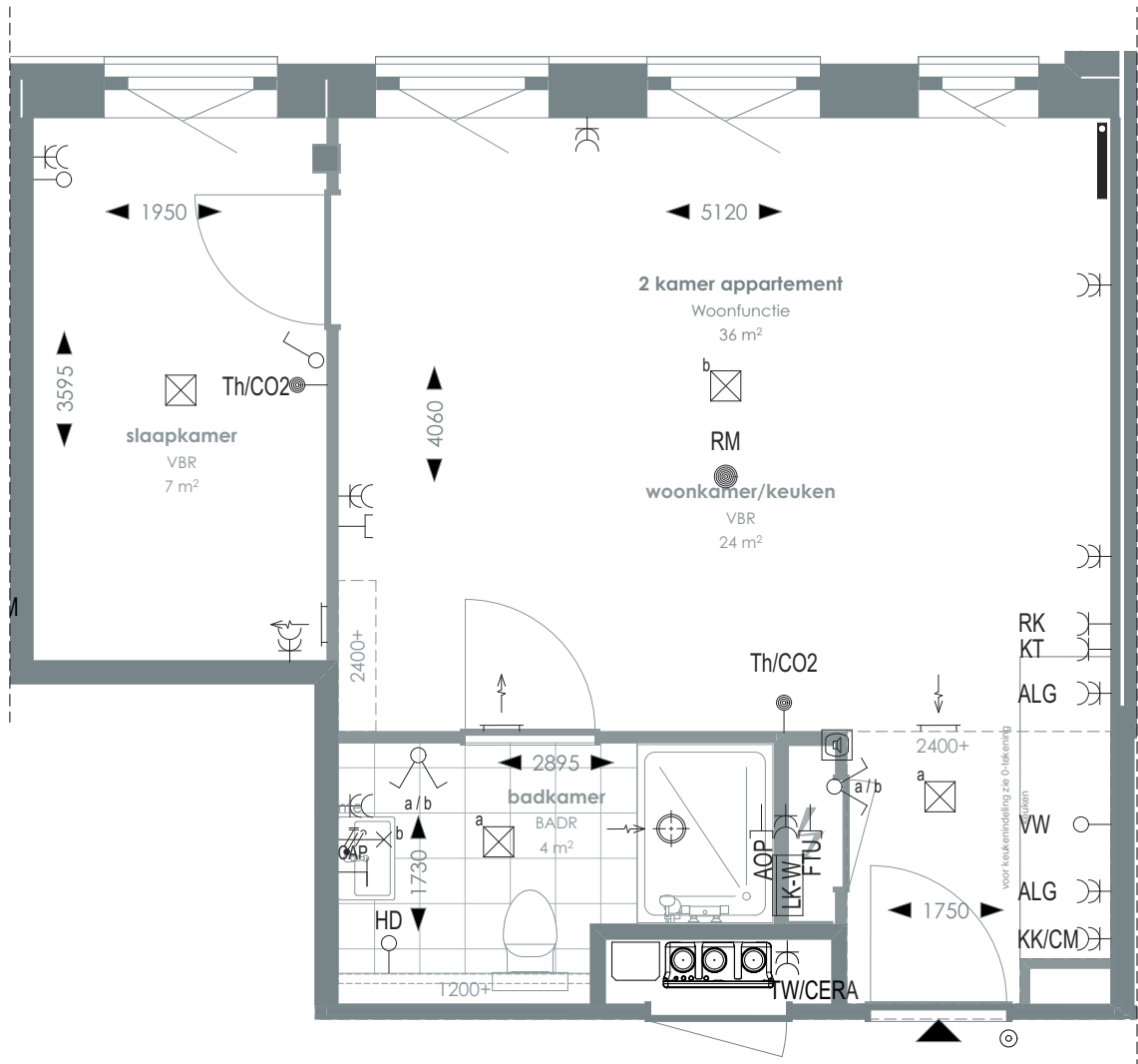
1:50 PLATTEGROND
