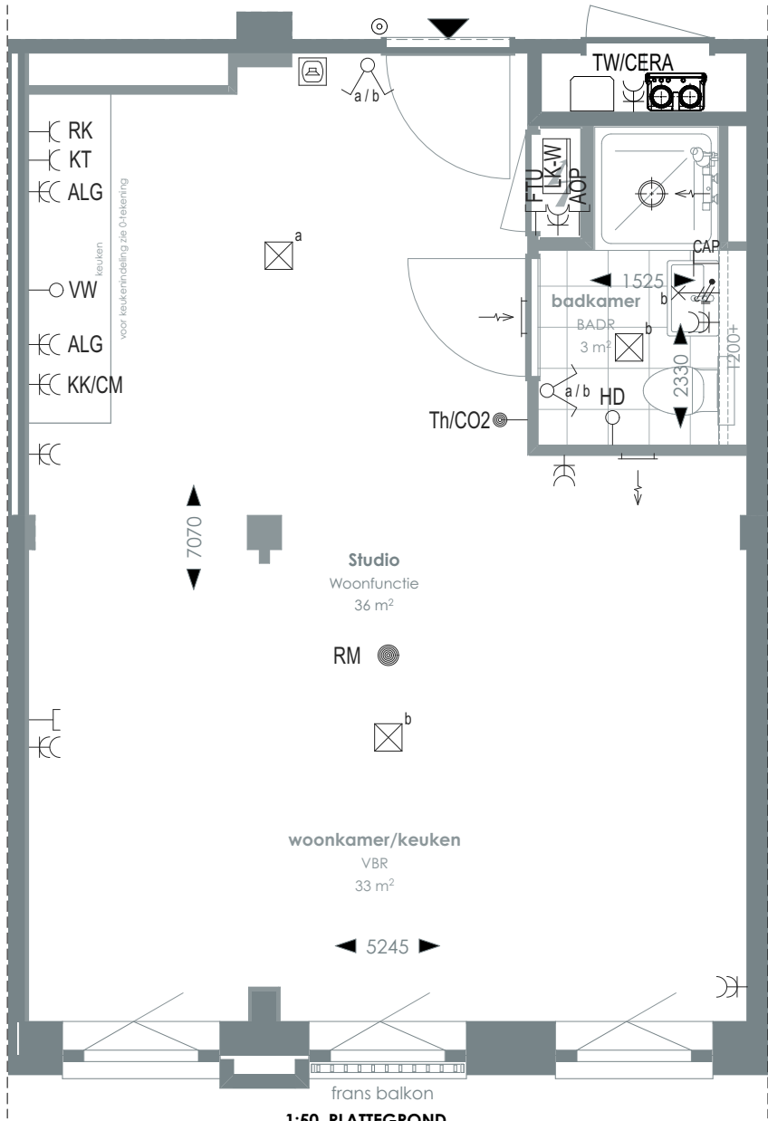
1:50 PLATTEGROND
