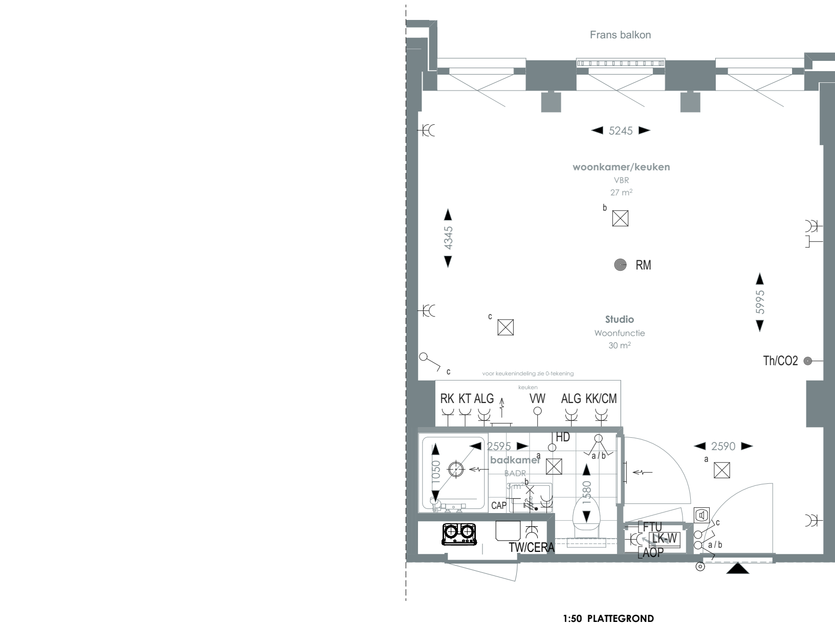
1:50 PLATTEGROND
