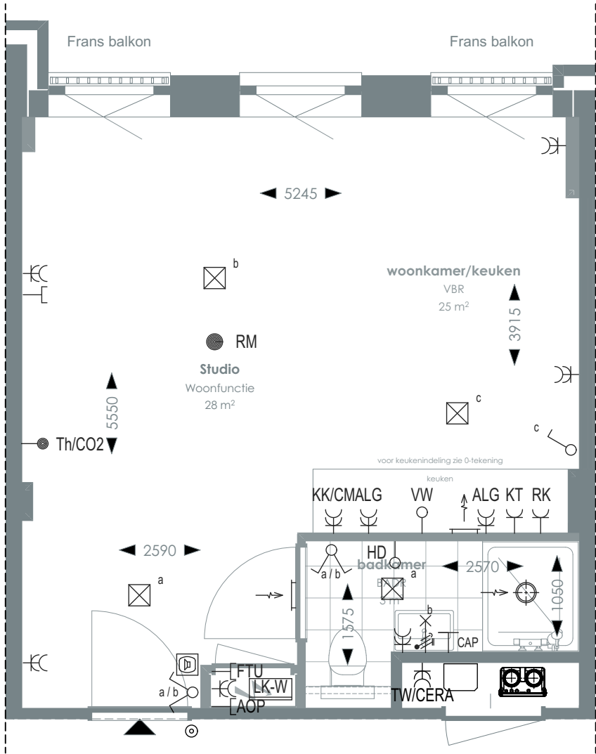
1:50 PLATTEGROND
