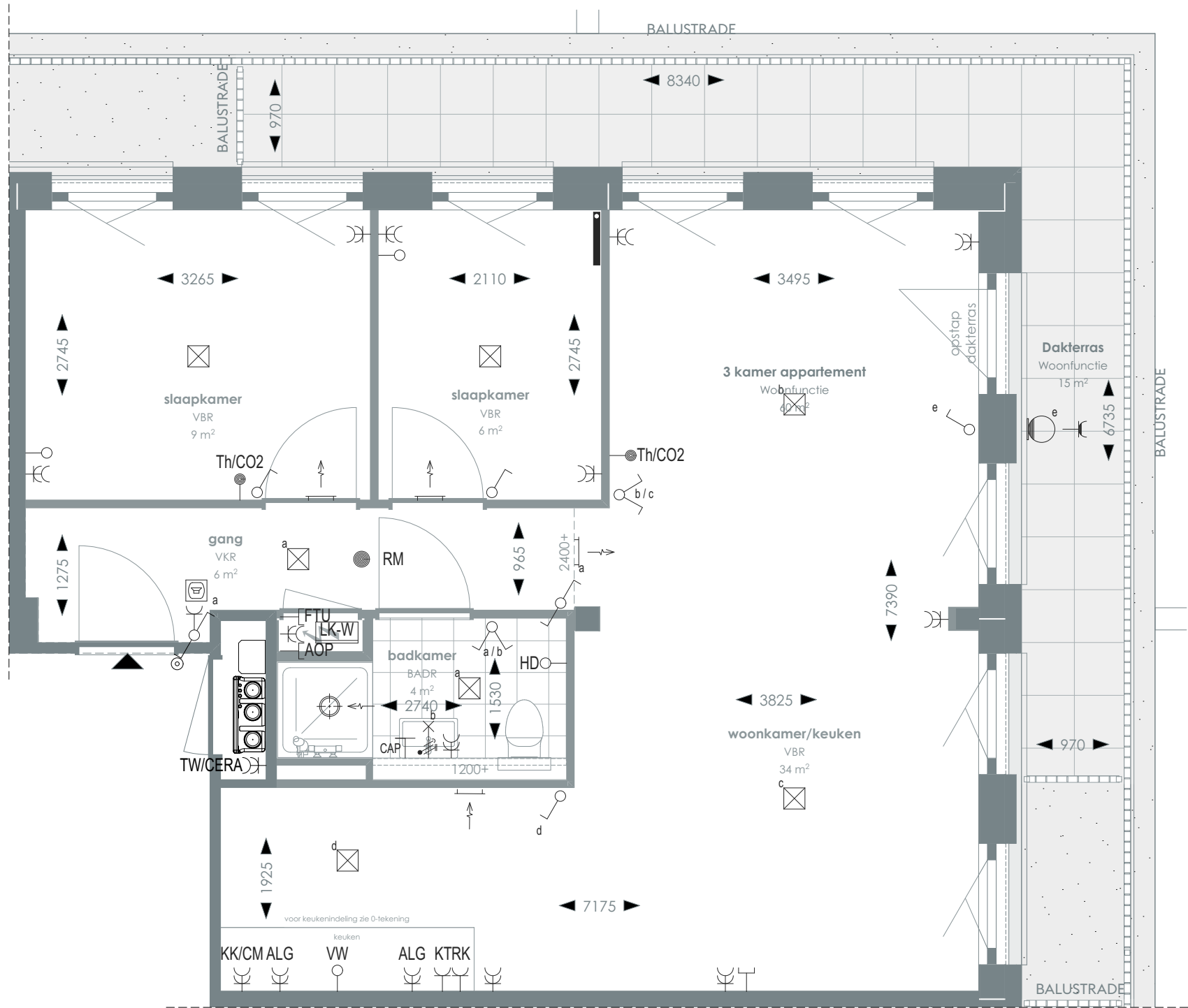
1:50 PLATTEGROND
