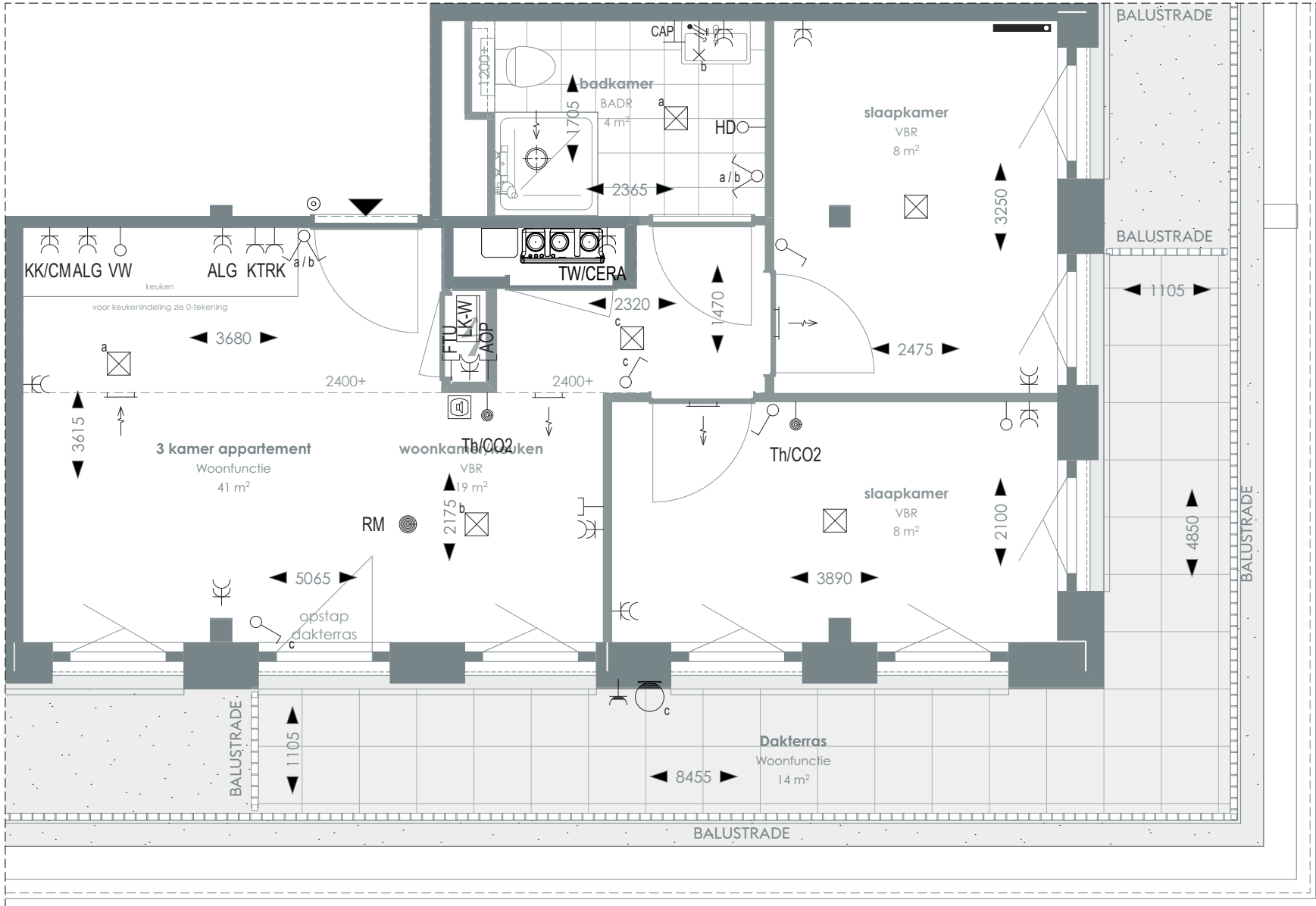
1:50 PLATTEGROND
