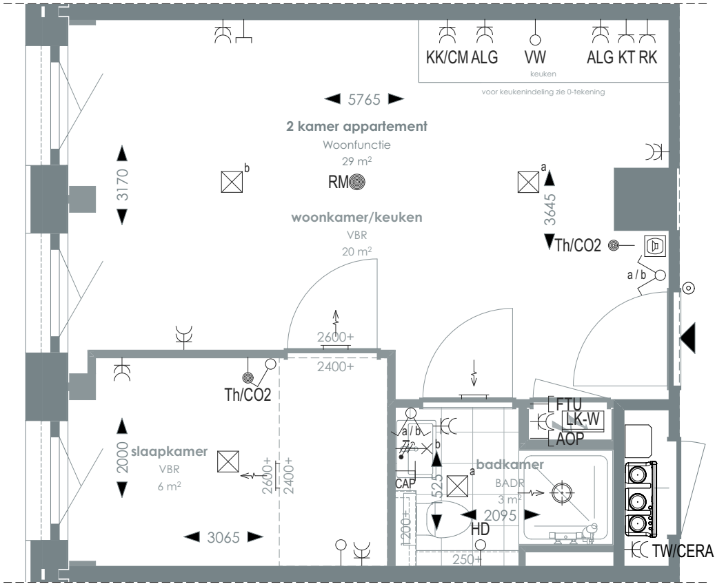
1:50 PLATTEGROND
