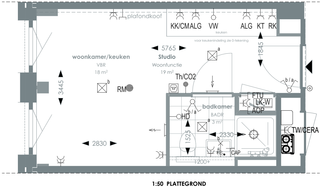
1:50 PLATTEGROND
