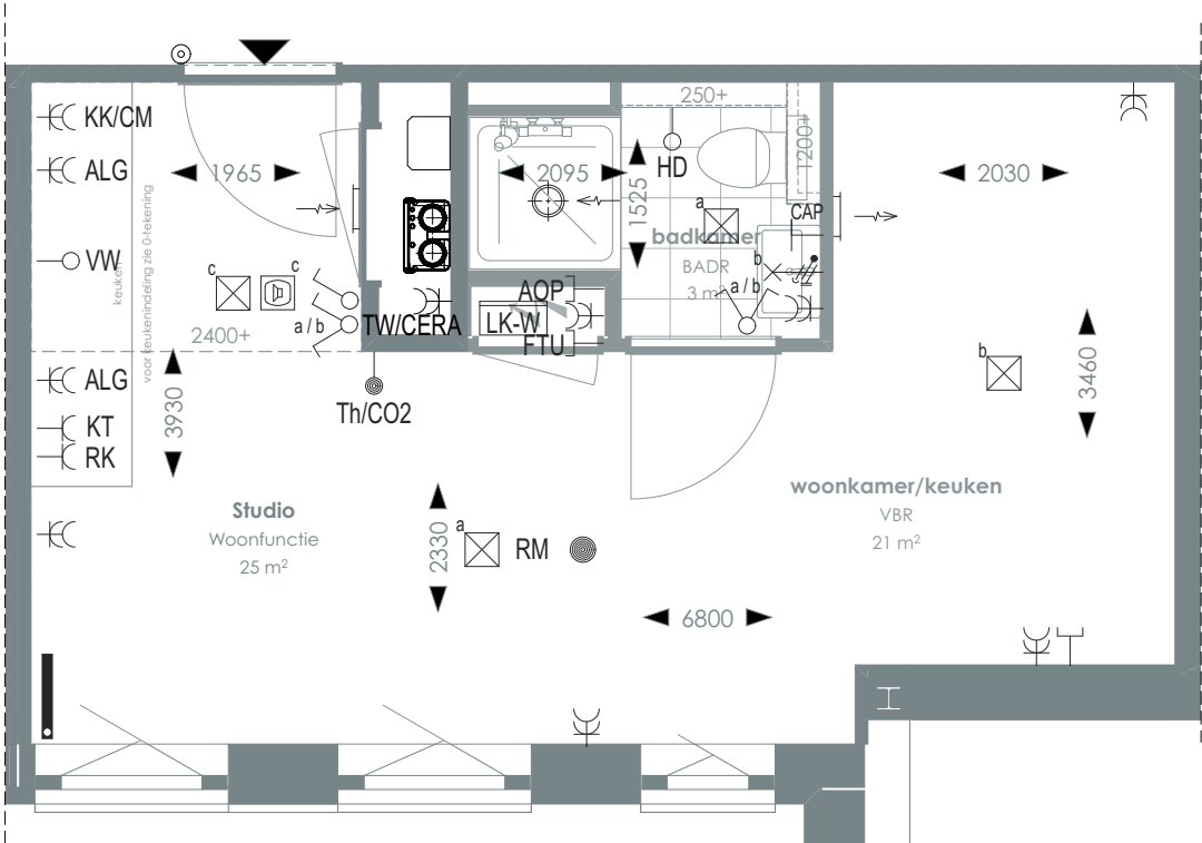
1:50 PLATTEGROND
