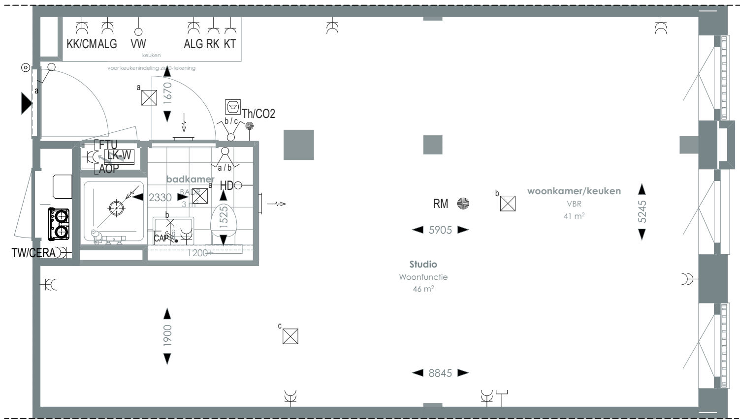
1:50 PLATTEGROND
