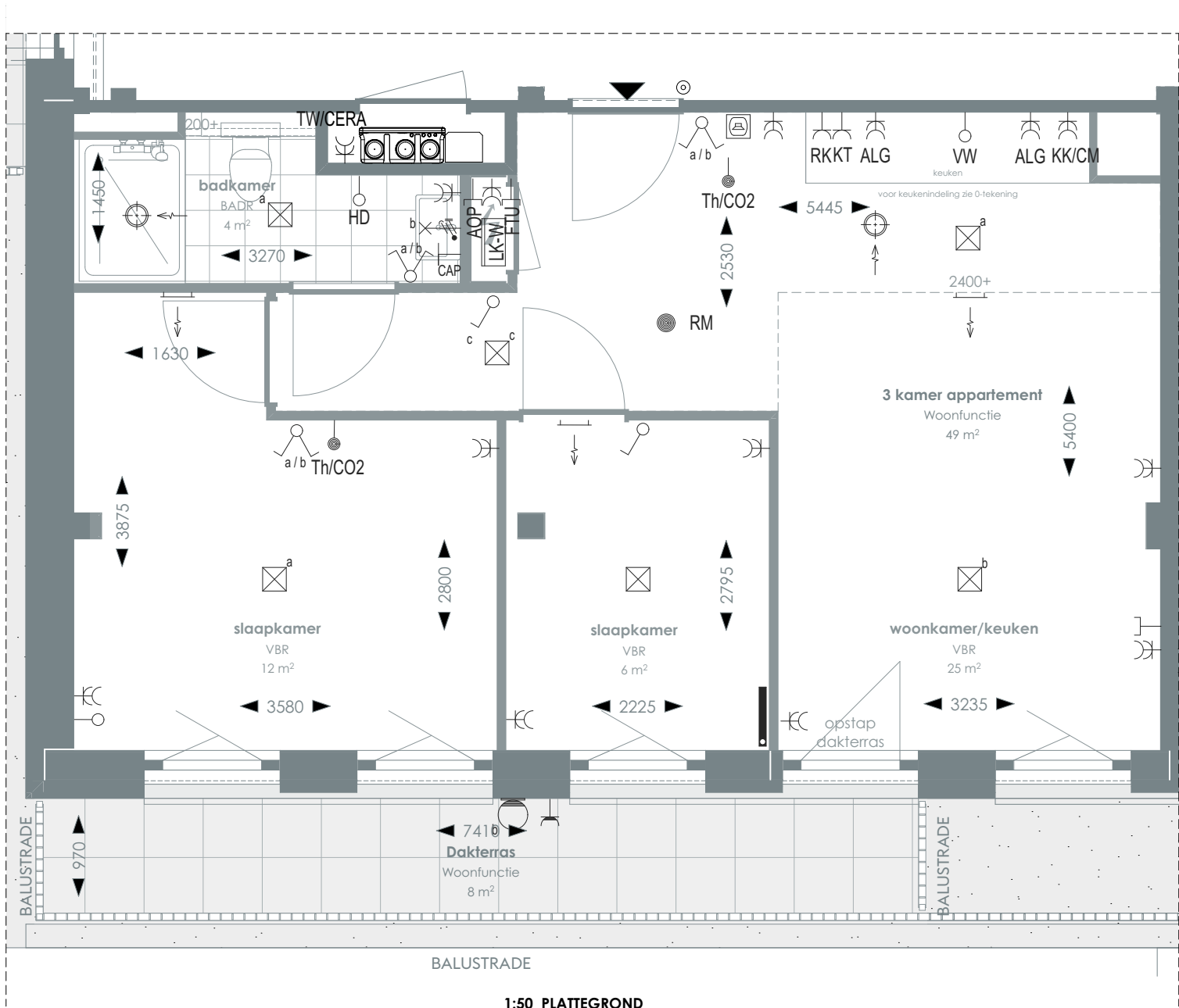
1:50 PLATTEGROND
