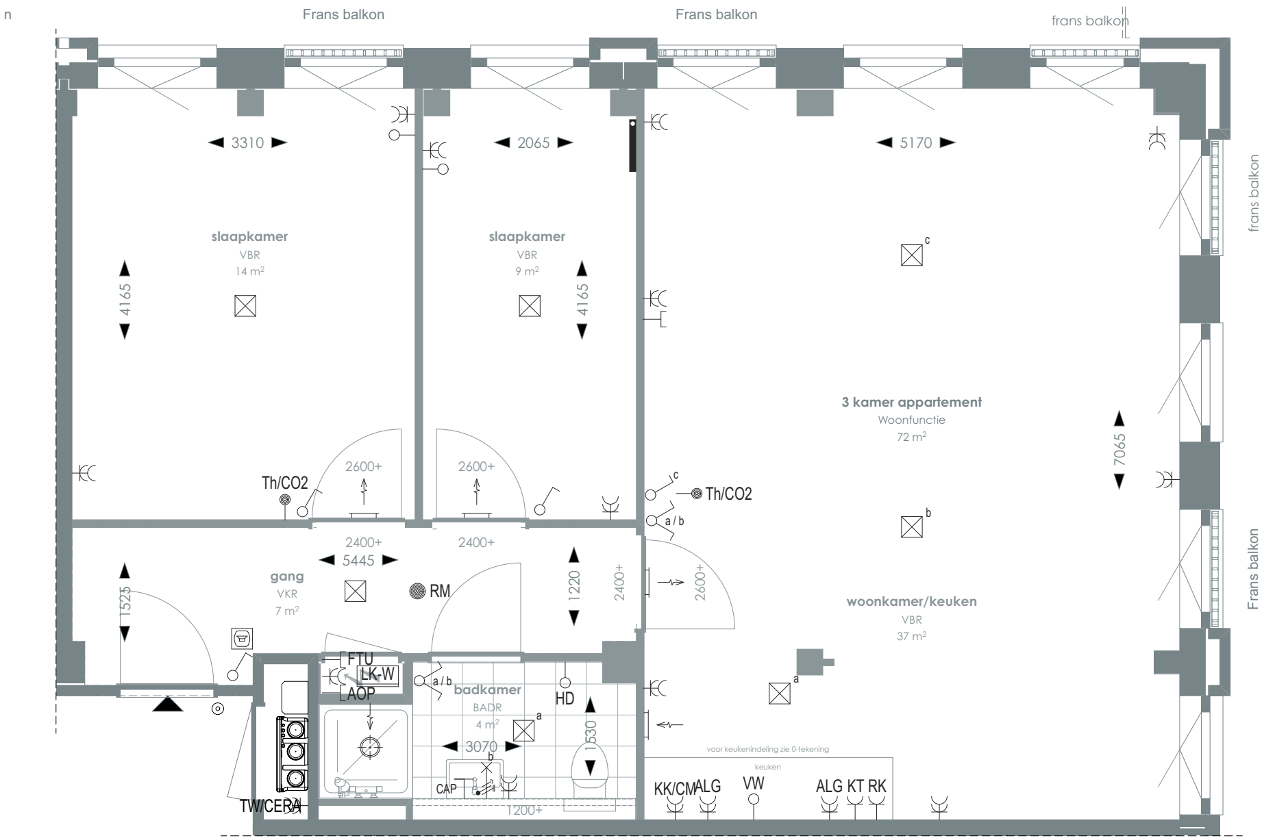
1:50 PLATTEGROND
