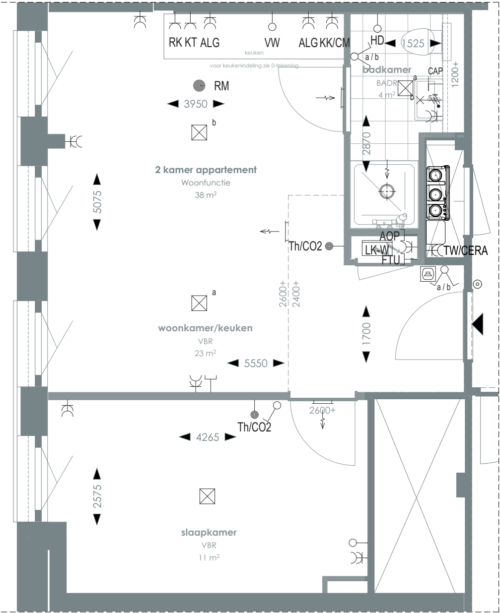
1:50 PLATTEGROND
