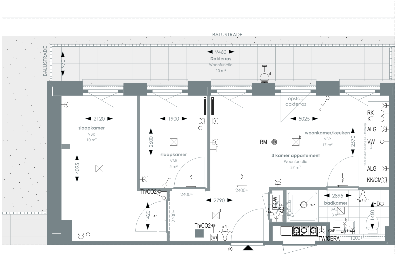
1:50 PLATTEGROND
