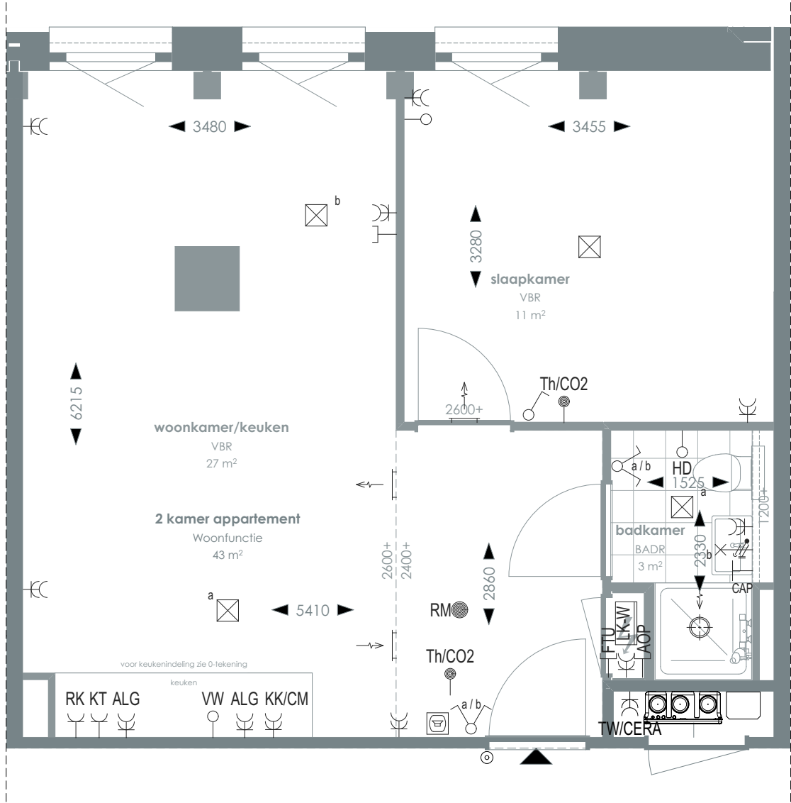
1:50 PLATTEGROND
