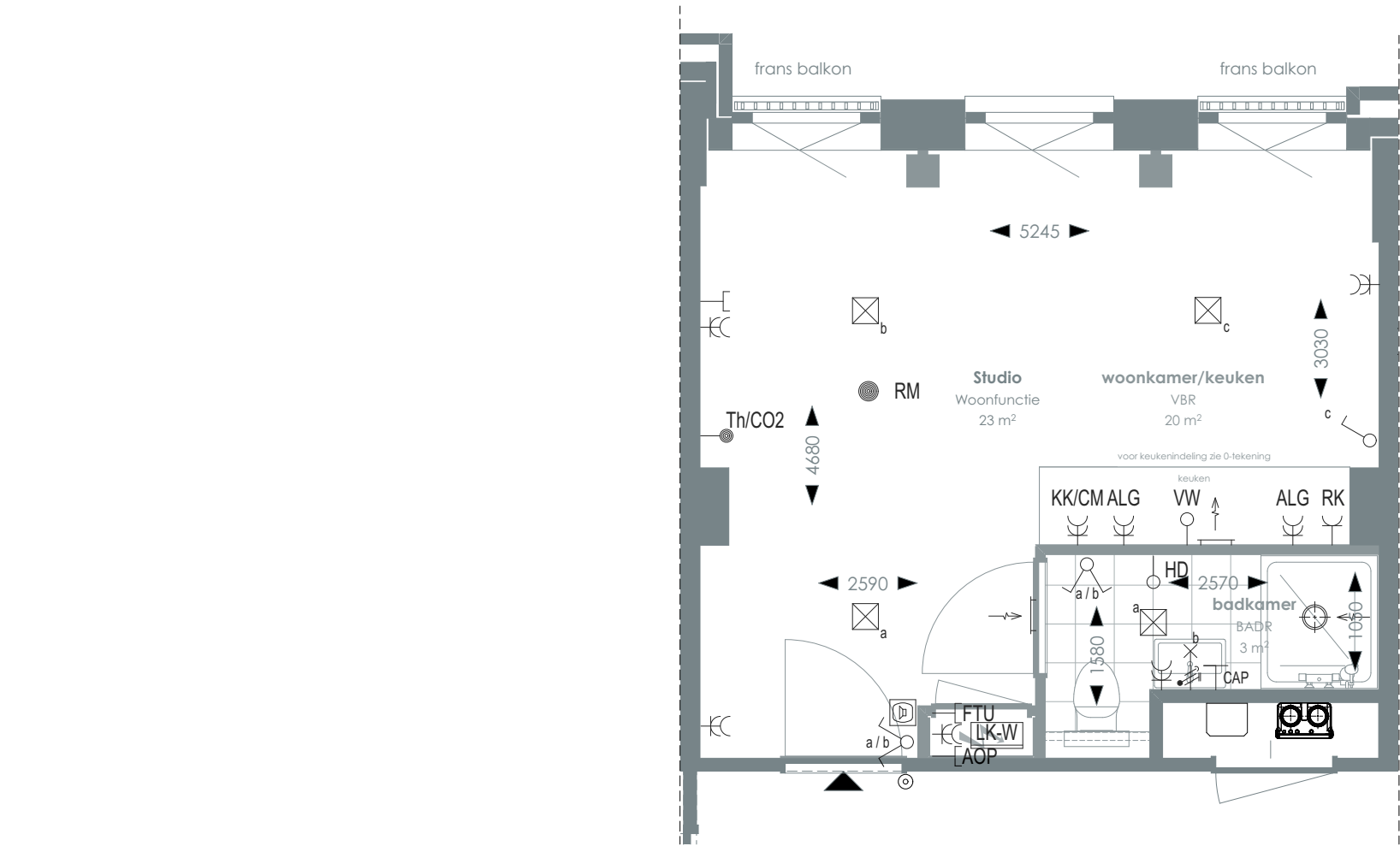
1:50 PLATTEGROND
