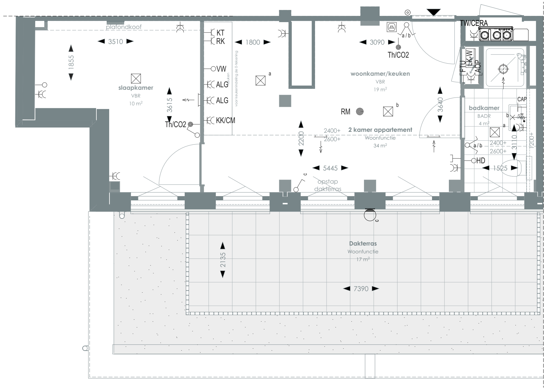
1:50 PLATTEGROND
