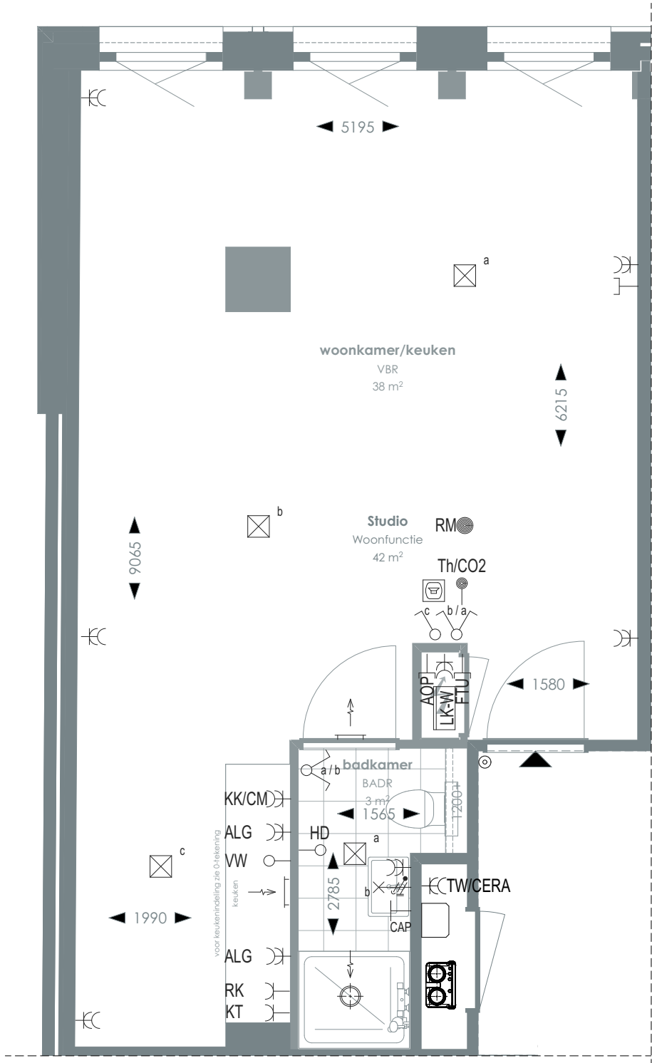
1:50 PLATTEGROND
