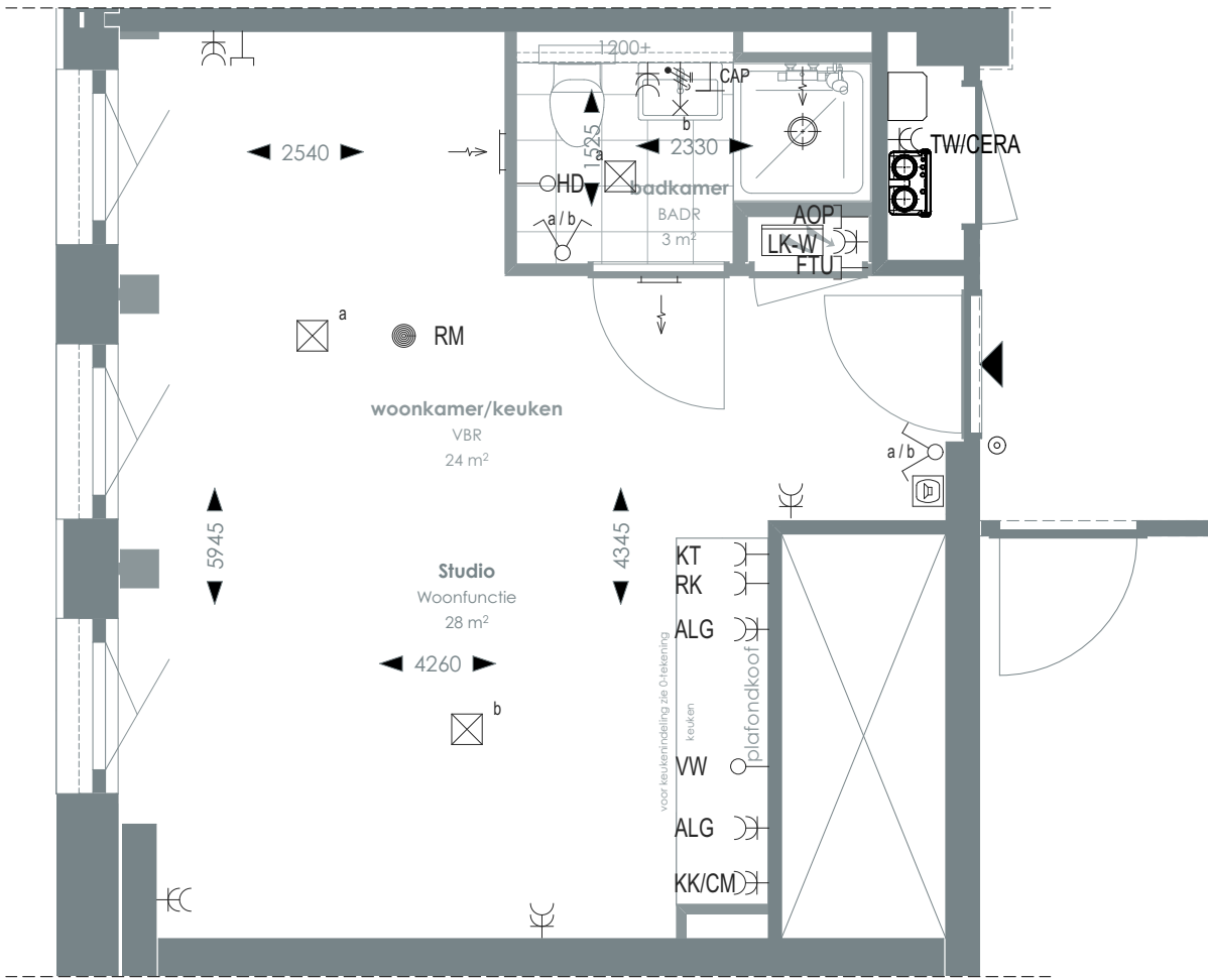
1:50 PLATTEGROND
