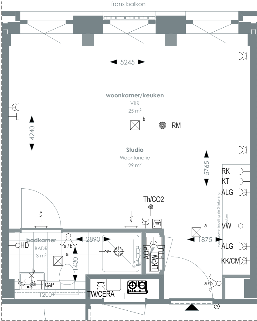
1:50 PLATTEGROND
