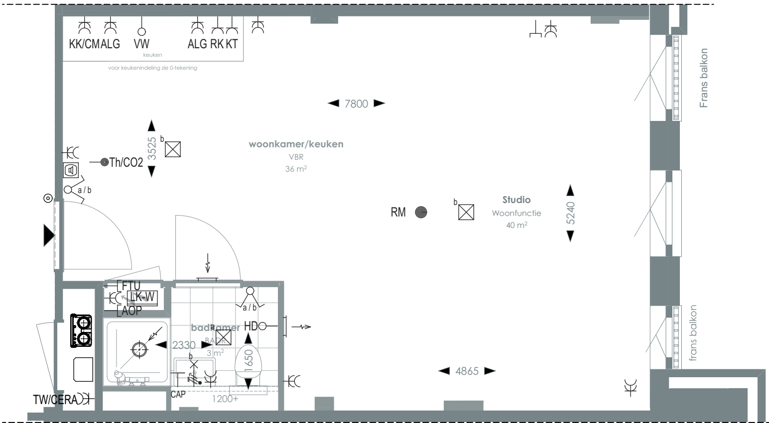
1:50 PLATTEGROND
