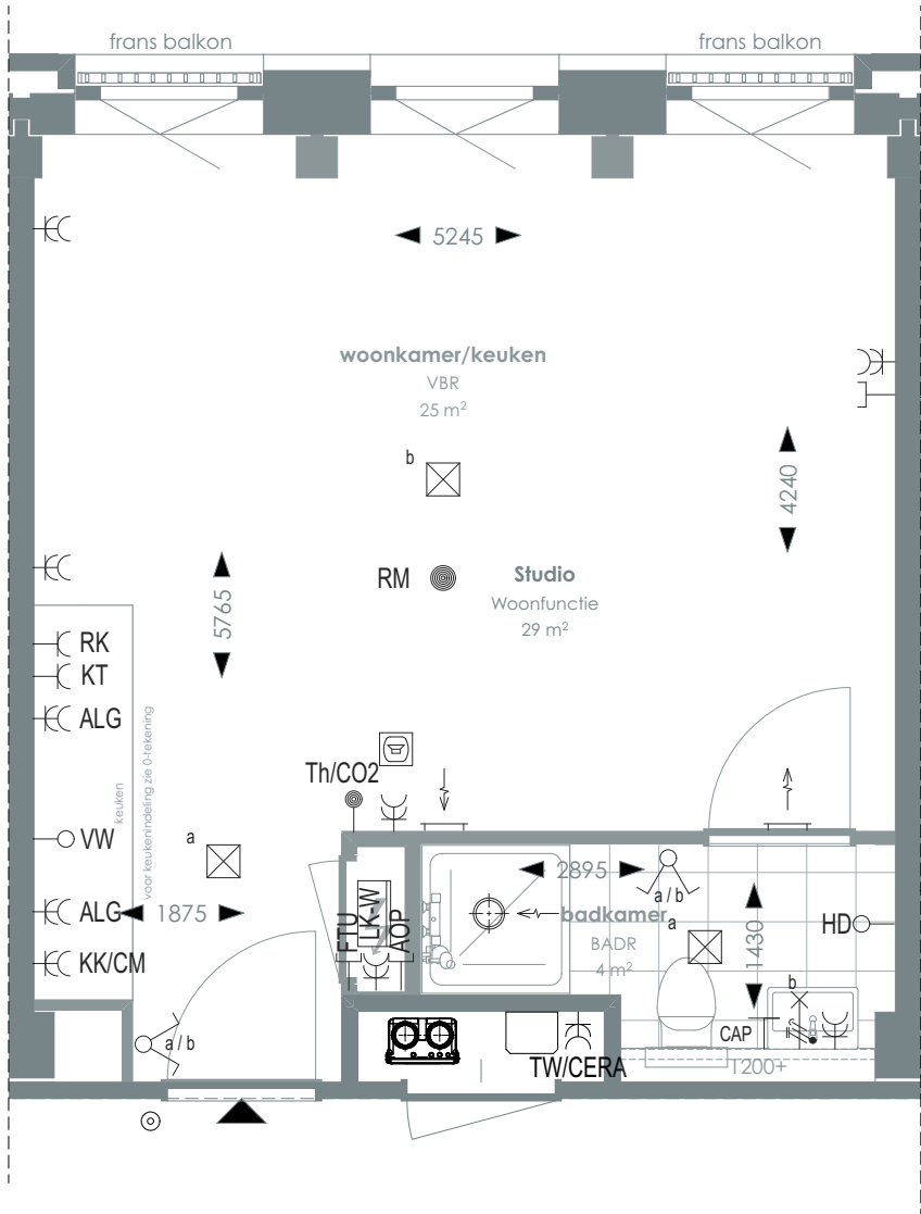
1:50 PLATTEGROND
