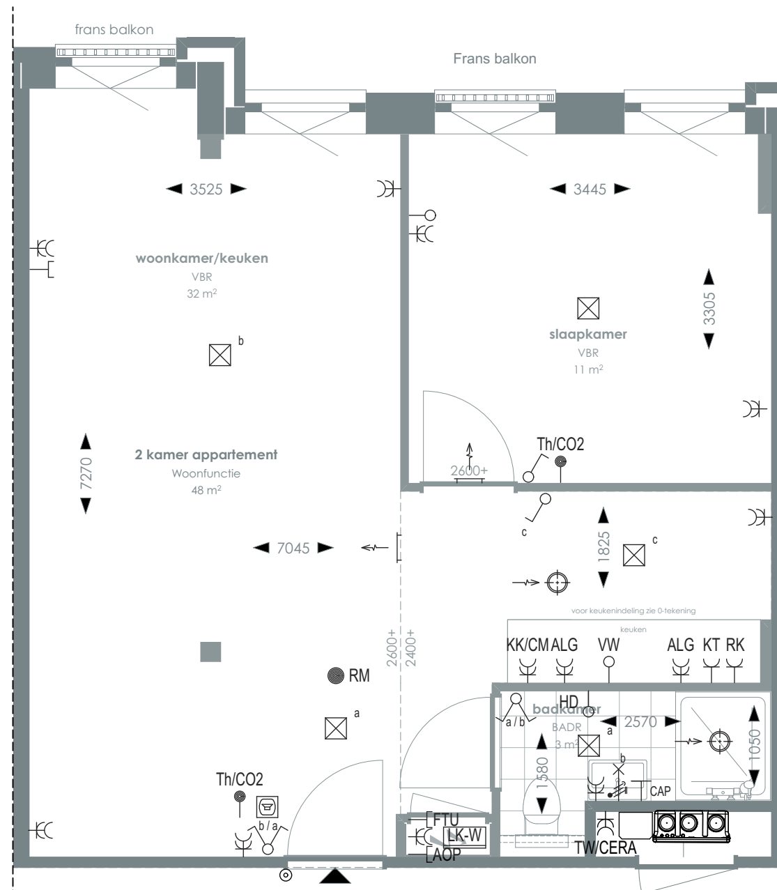
1:50 PLATTEGROND
