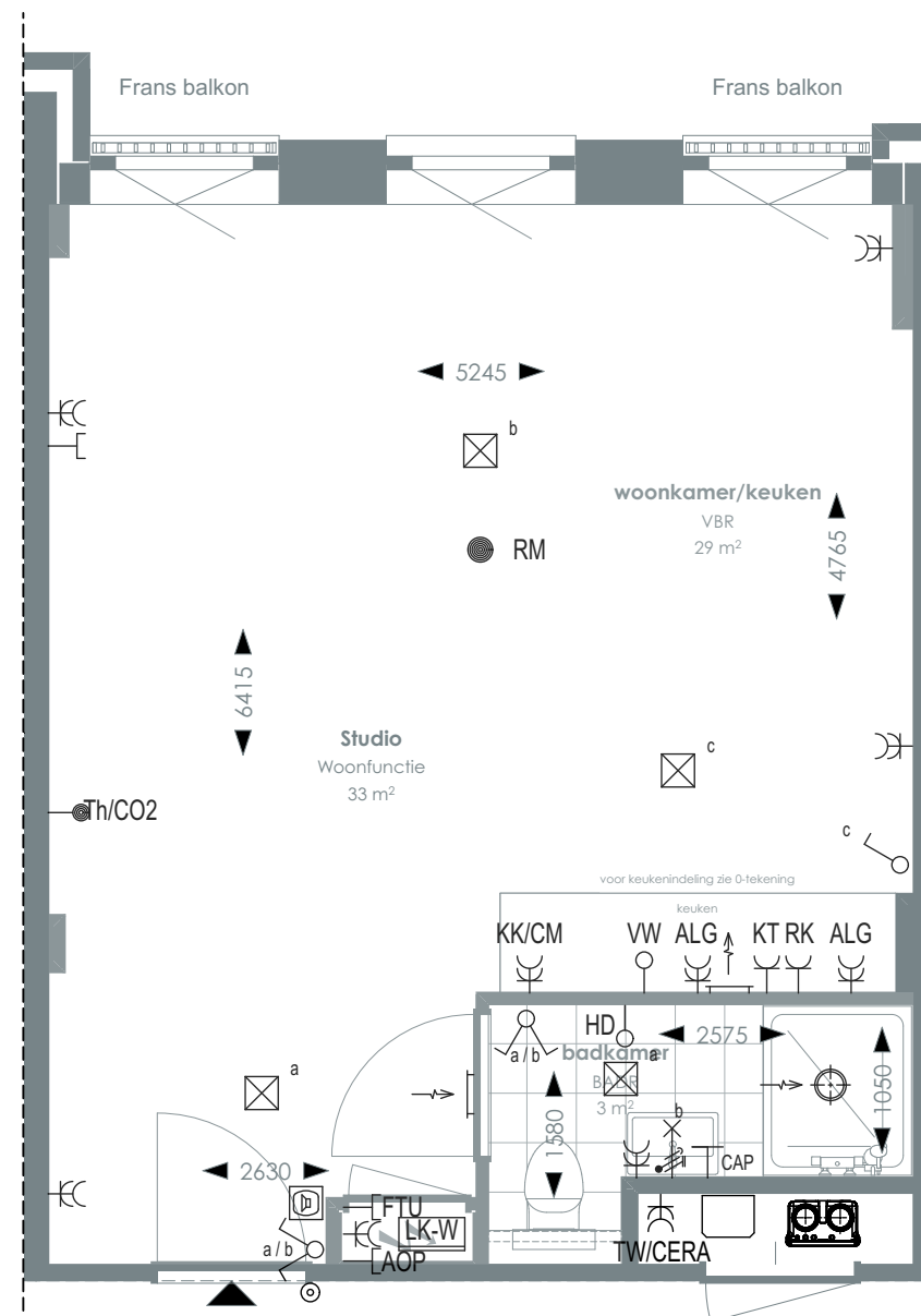
1:50 PLATTEGROND
