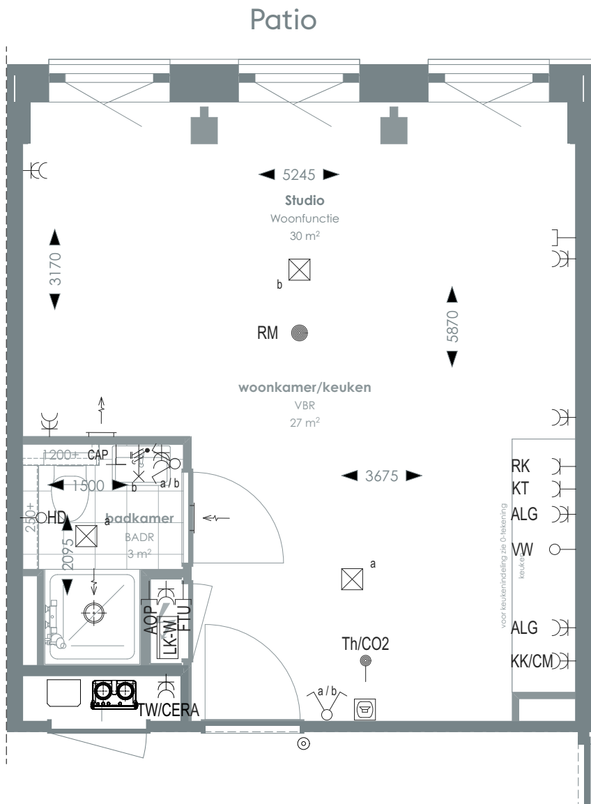
1:50 PLATTEGROND
