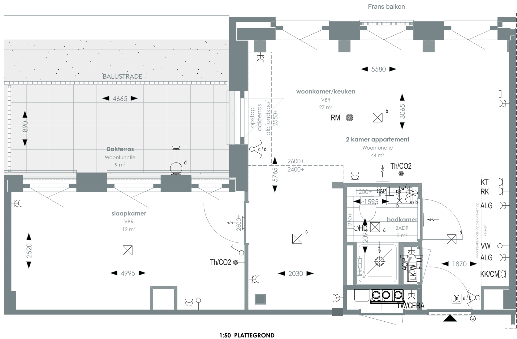
1:50 PLATTEGROND
