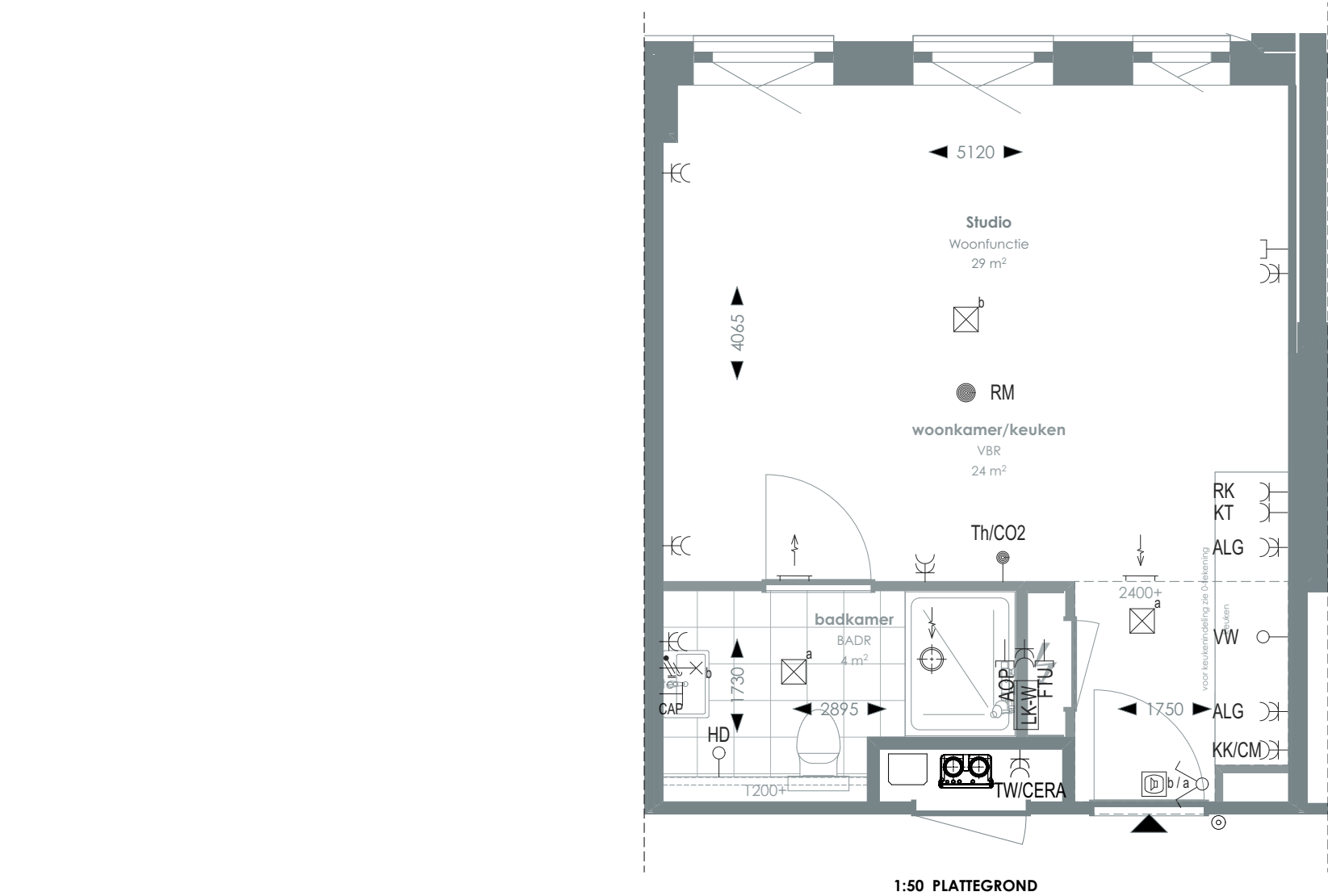
1:50 PLATTEGROND
