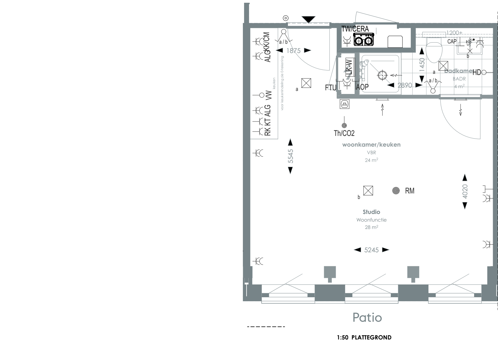
1:50 PLATTEGROND
