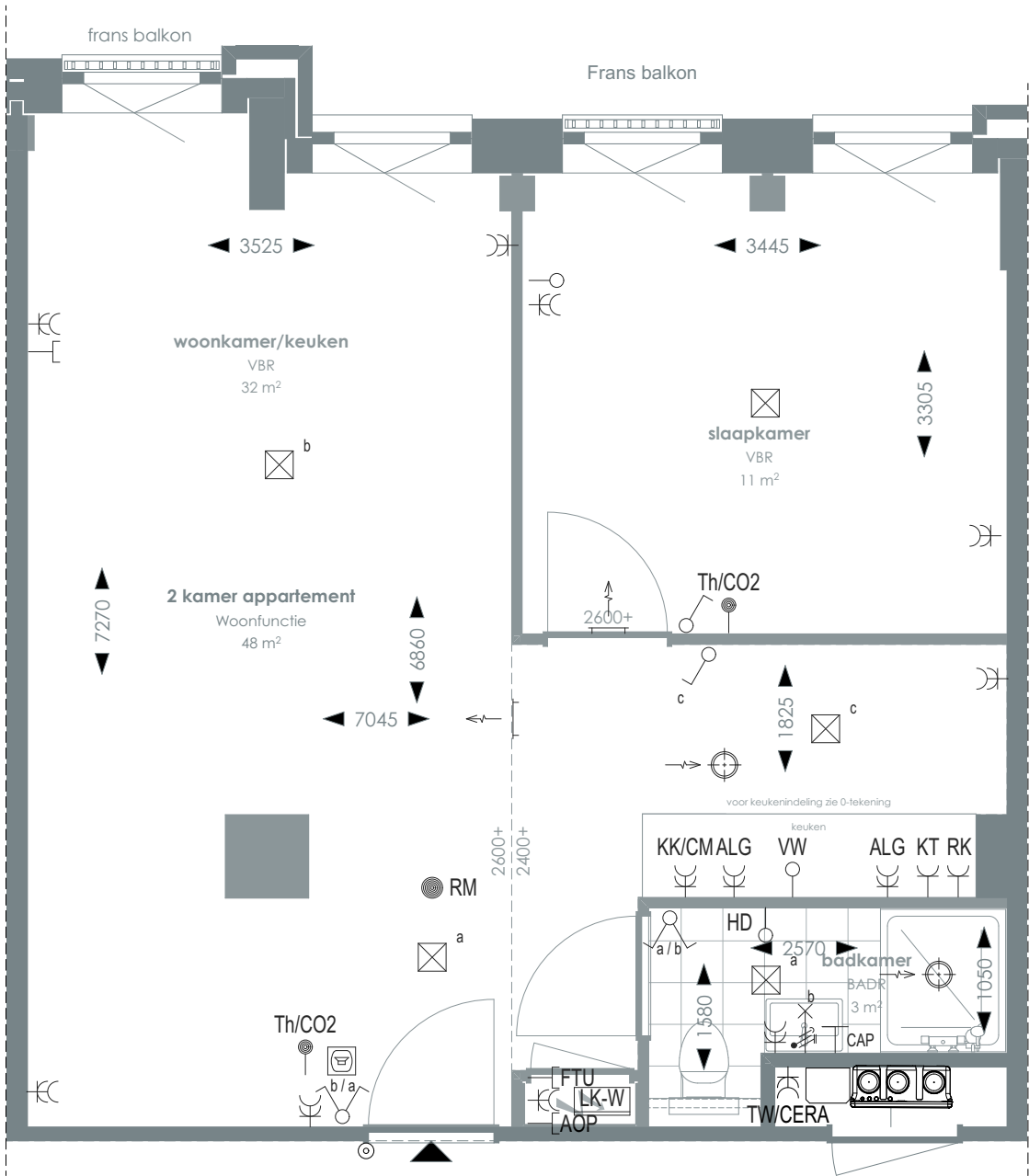
1:50 PLATTEGROND
