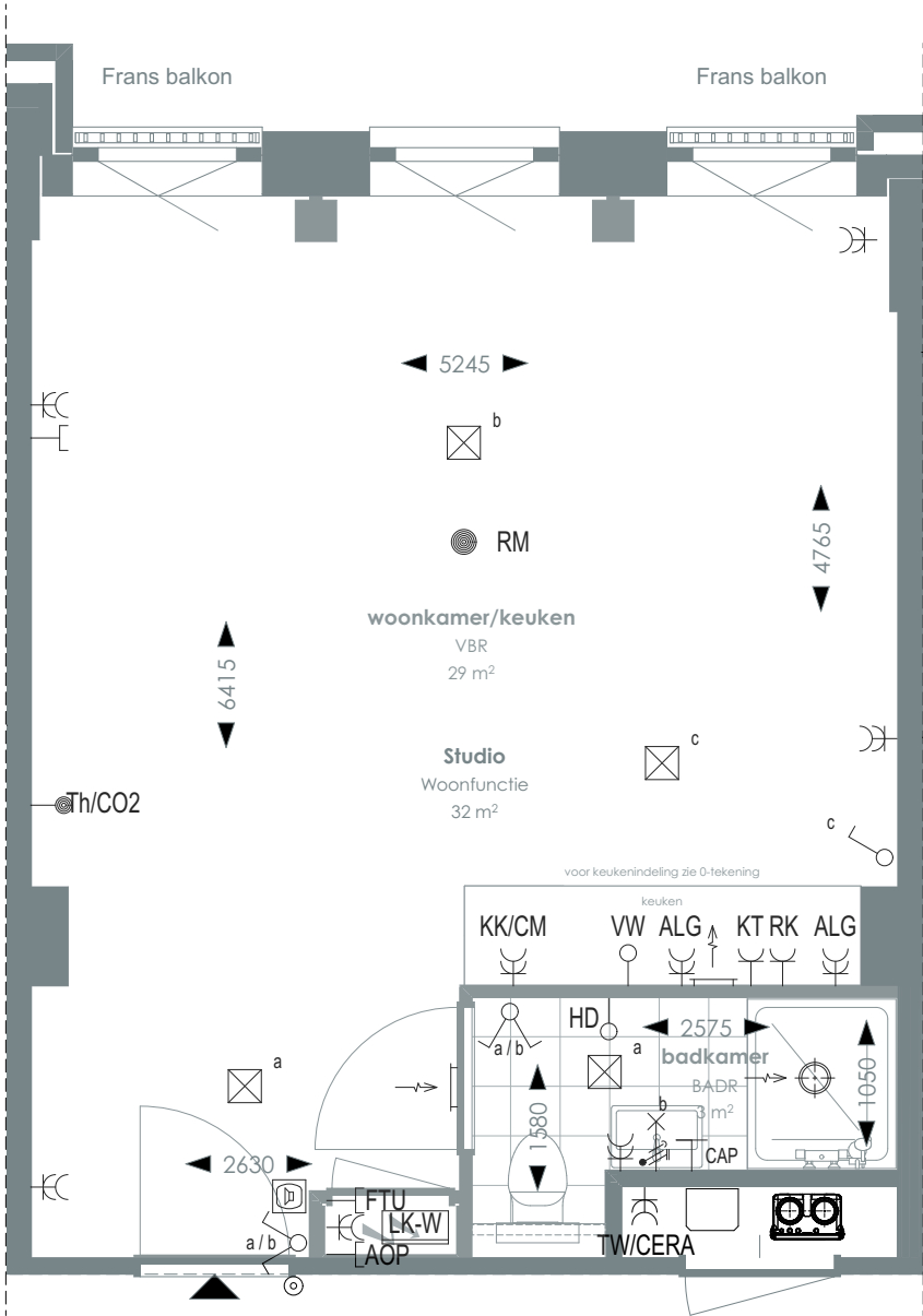
1:50 PLATTEGROND
