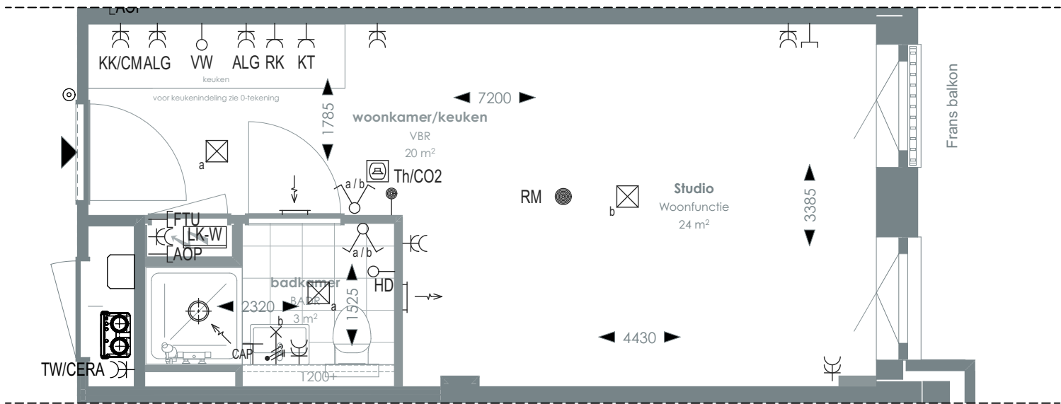
1:50 PLATTEGROND
