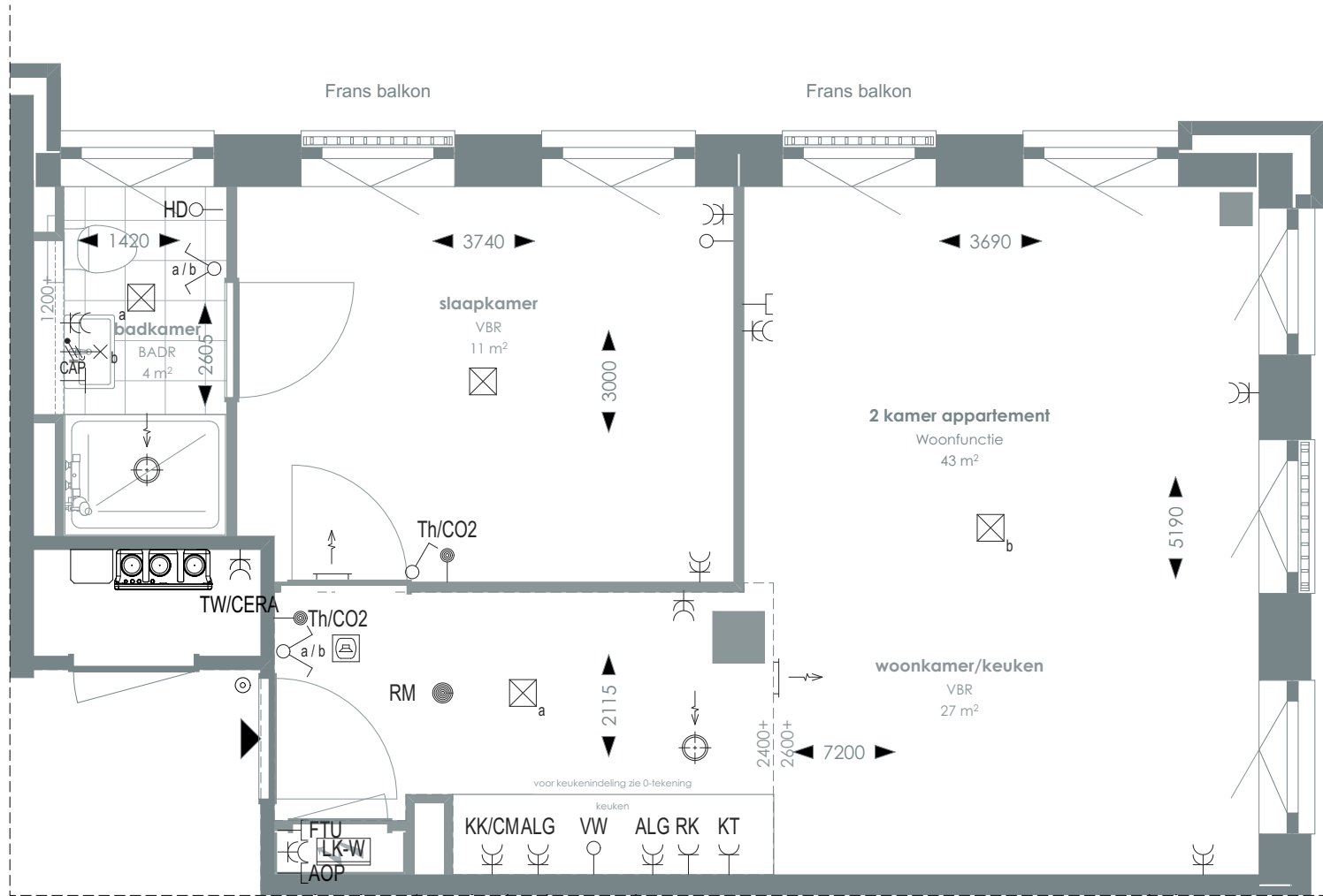
1:50 PLATTEGROND
