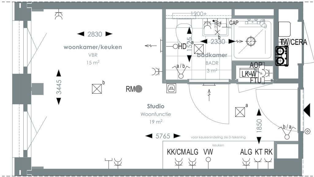
1:50 PLATTEGROND
