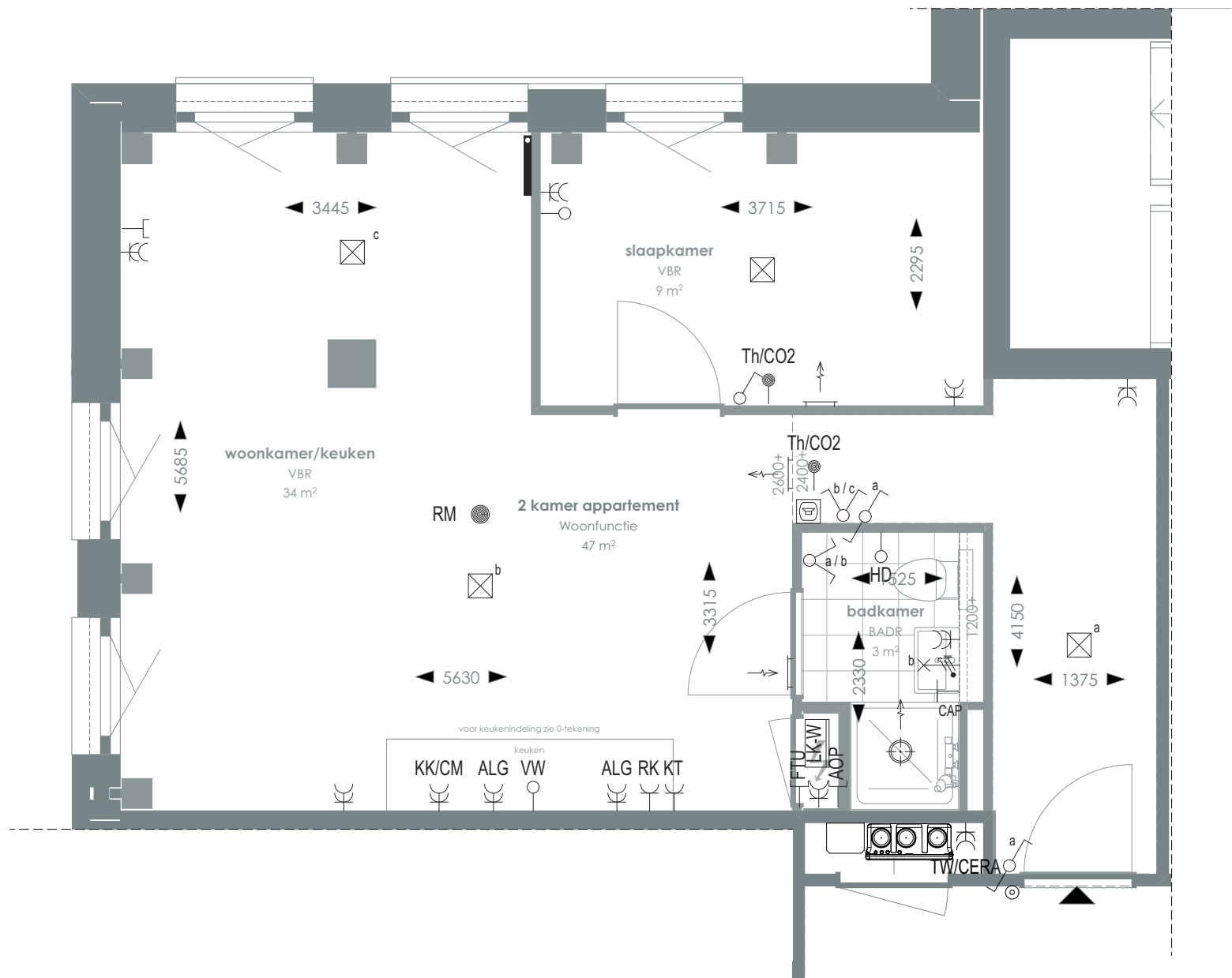
1:50 PLATTEGROND
