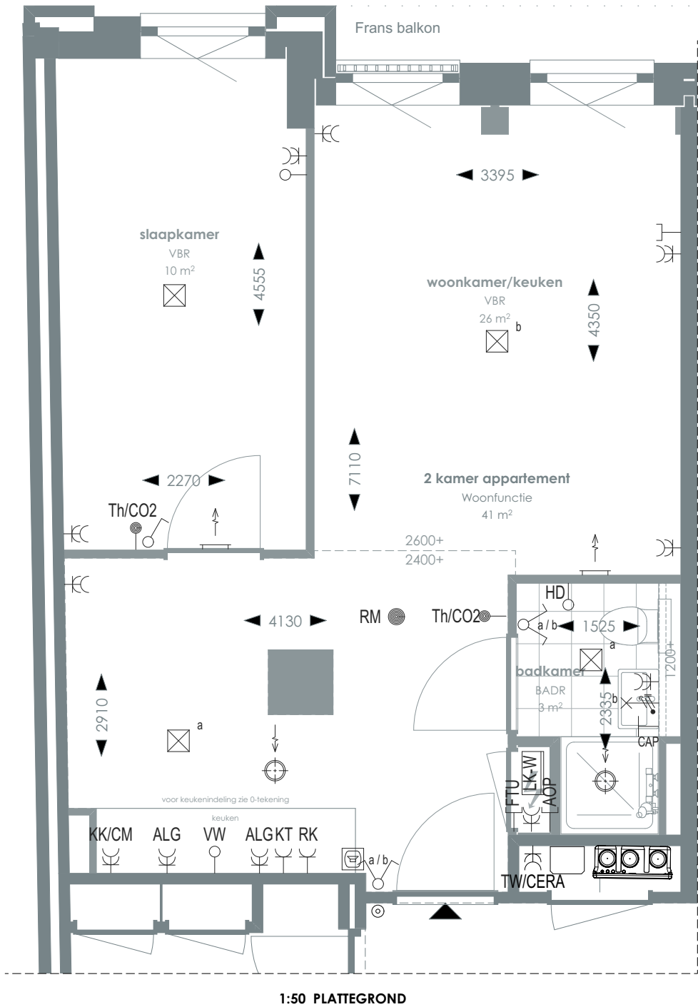
1:50 PLATTEGROND
