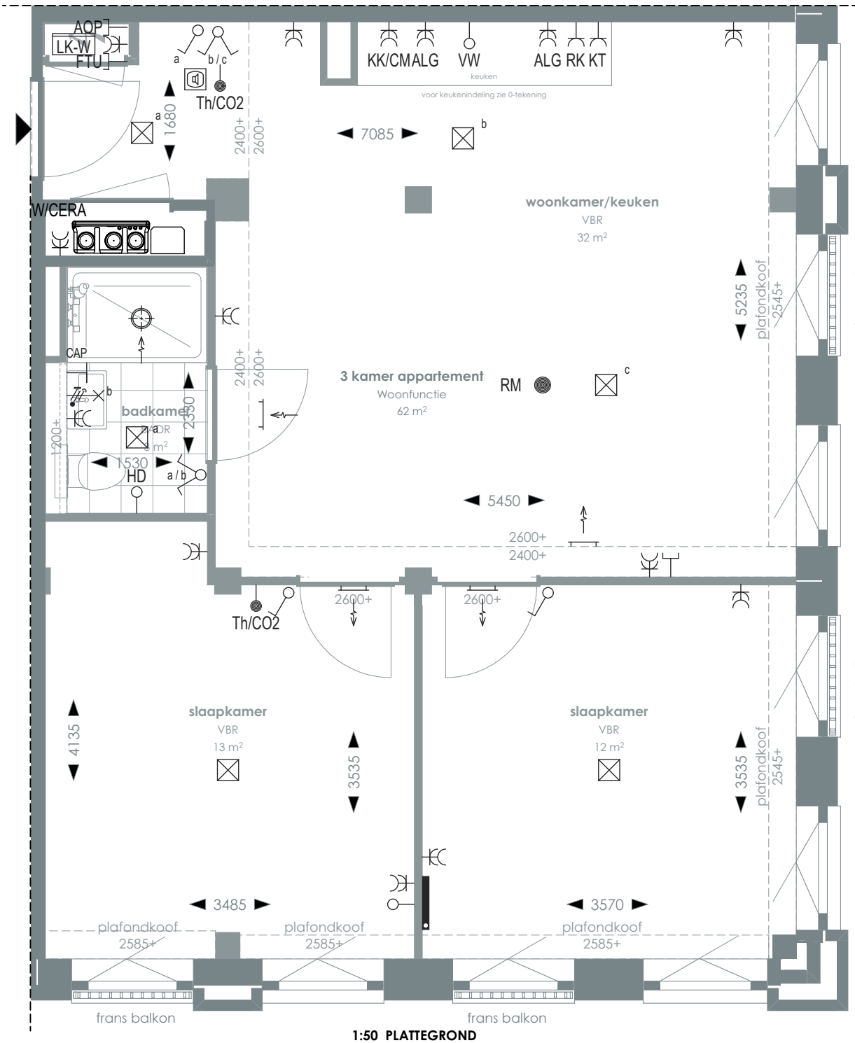
1:50 PLATTEGROND
