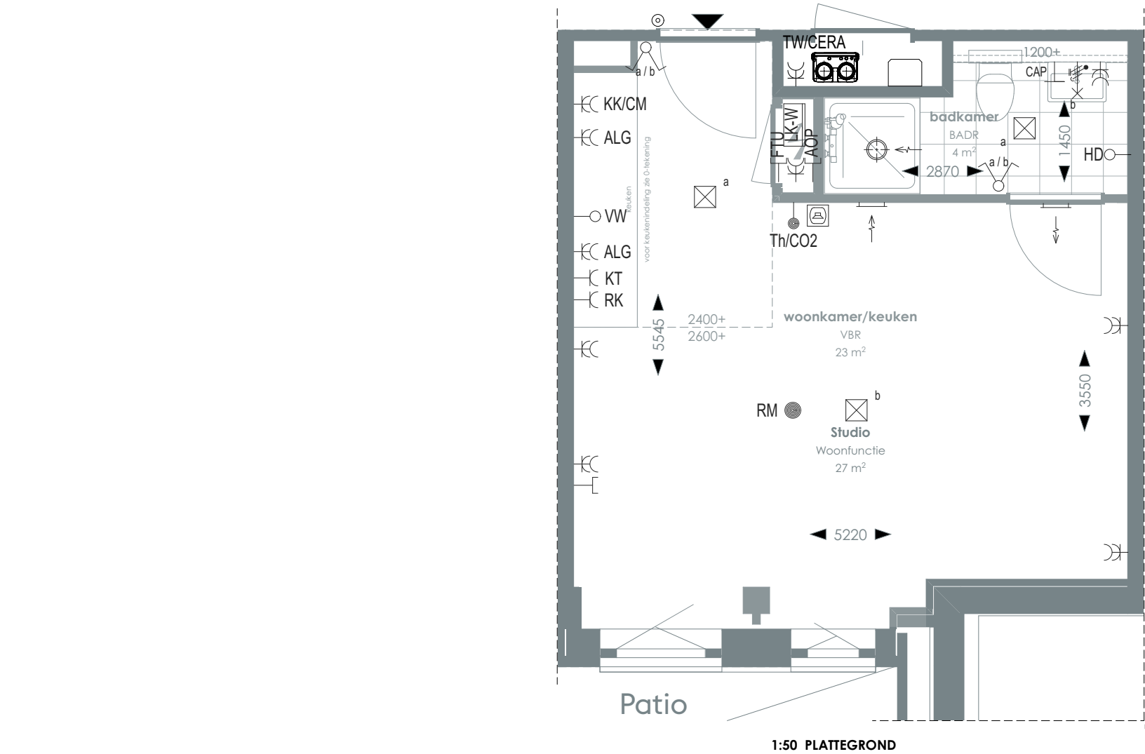
1:50 PLATTEGROND
