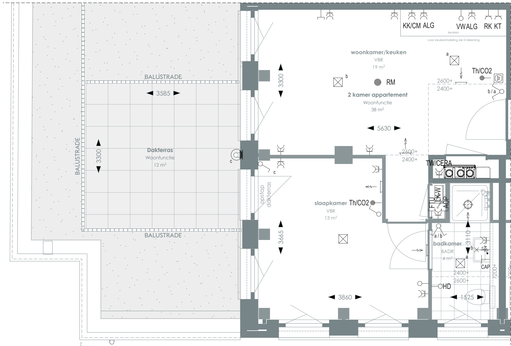
1:50 PLATTEGROND
