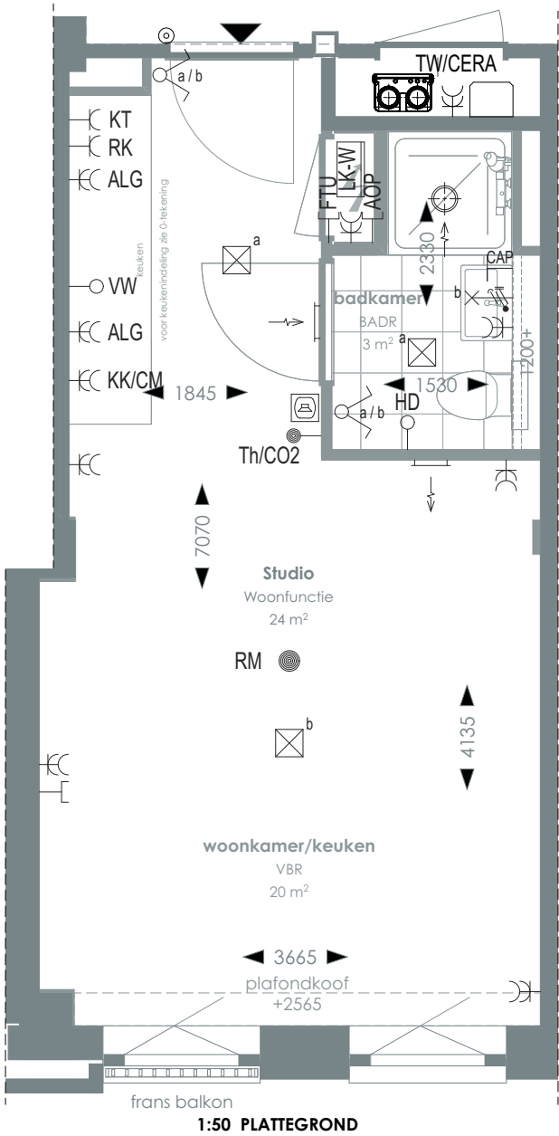
1:50 PLATTEGROND
