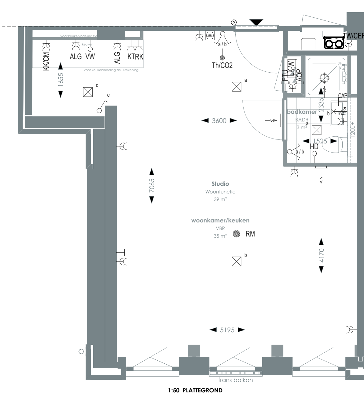
1:50 PLATTEGROND
