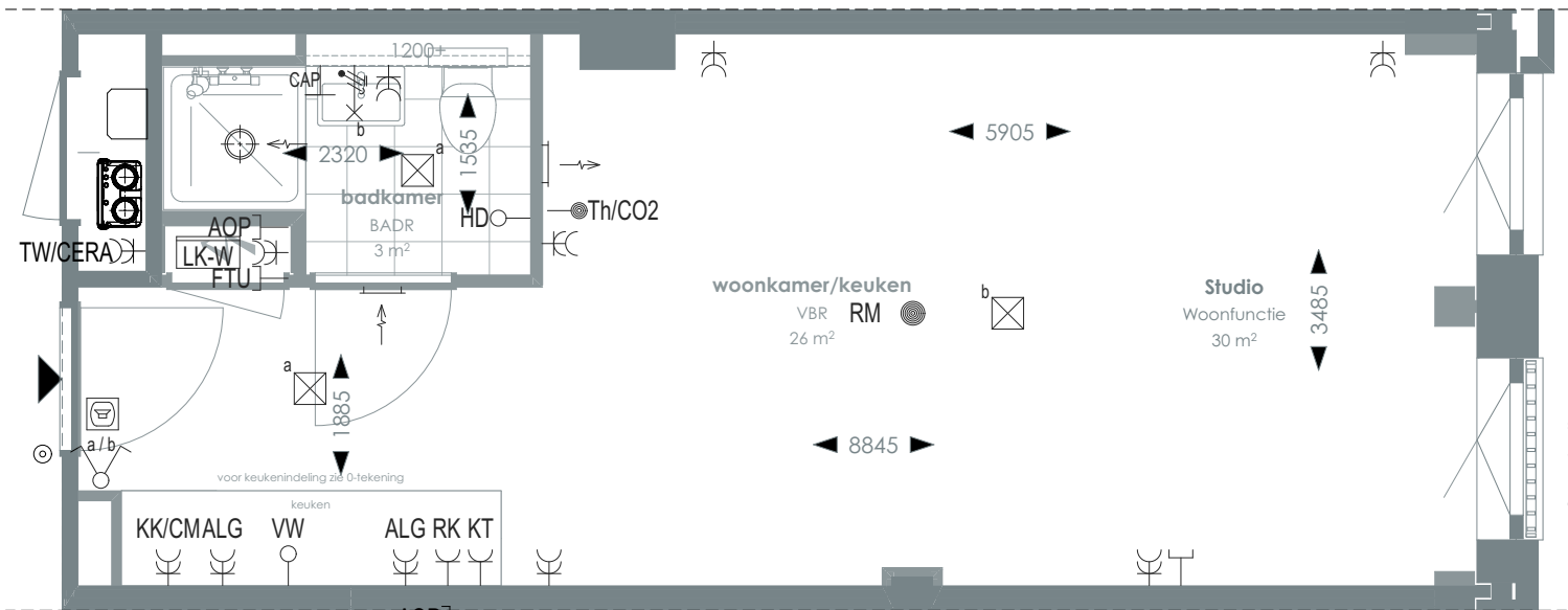
1:50 PLATTEGROND
