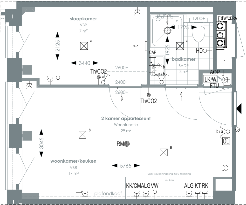
1:50 PLATTEGROND
