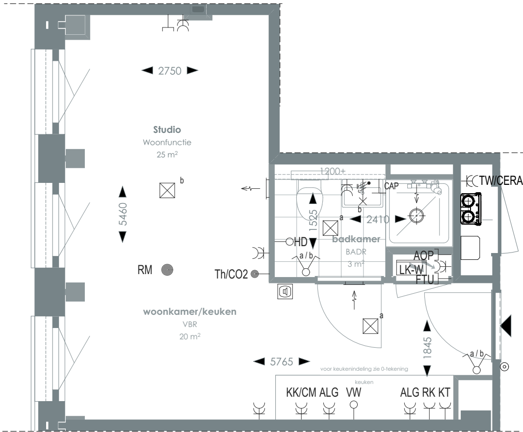
1:50 PLATTEGROND
