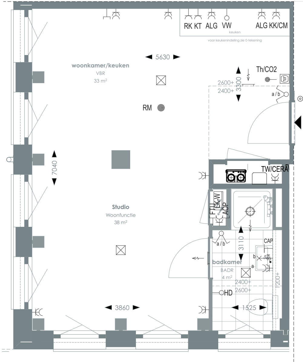
1:50 PLATTEGROND
