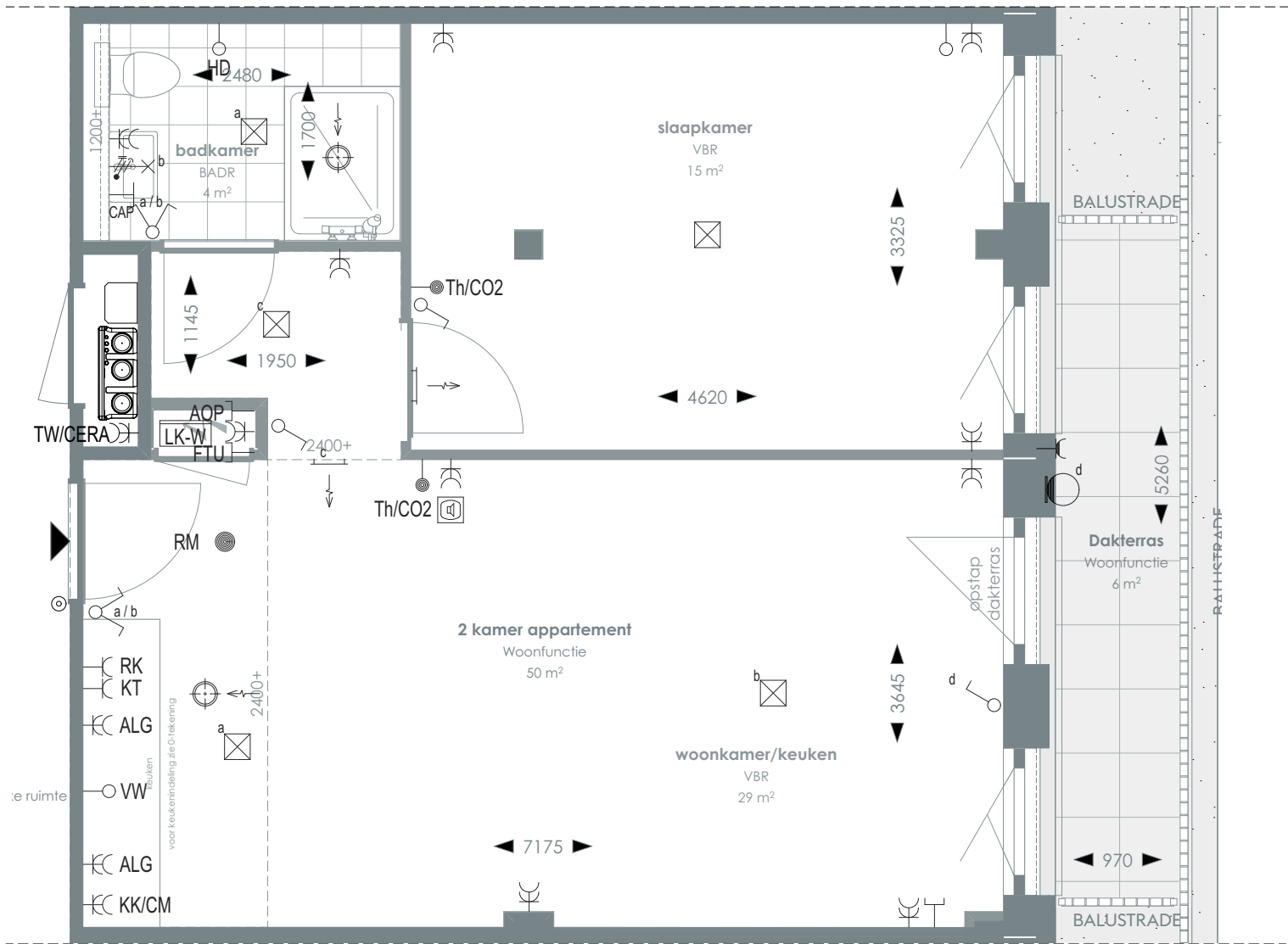
1:50 PLATTEGROND
