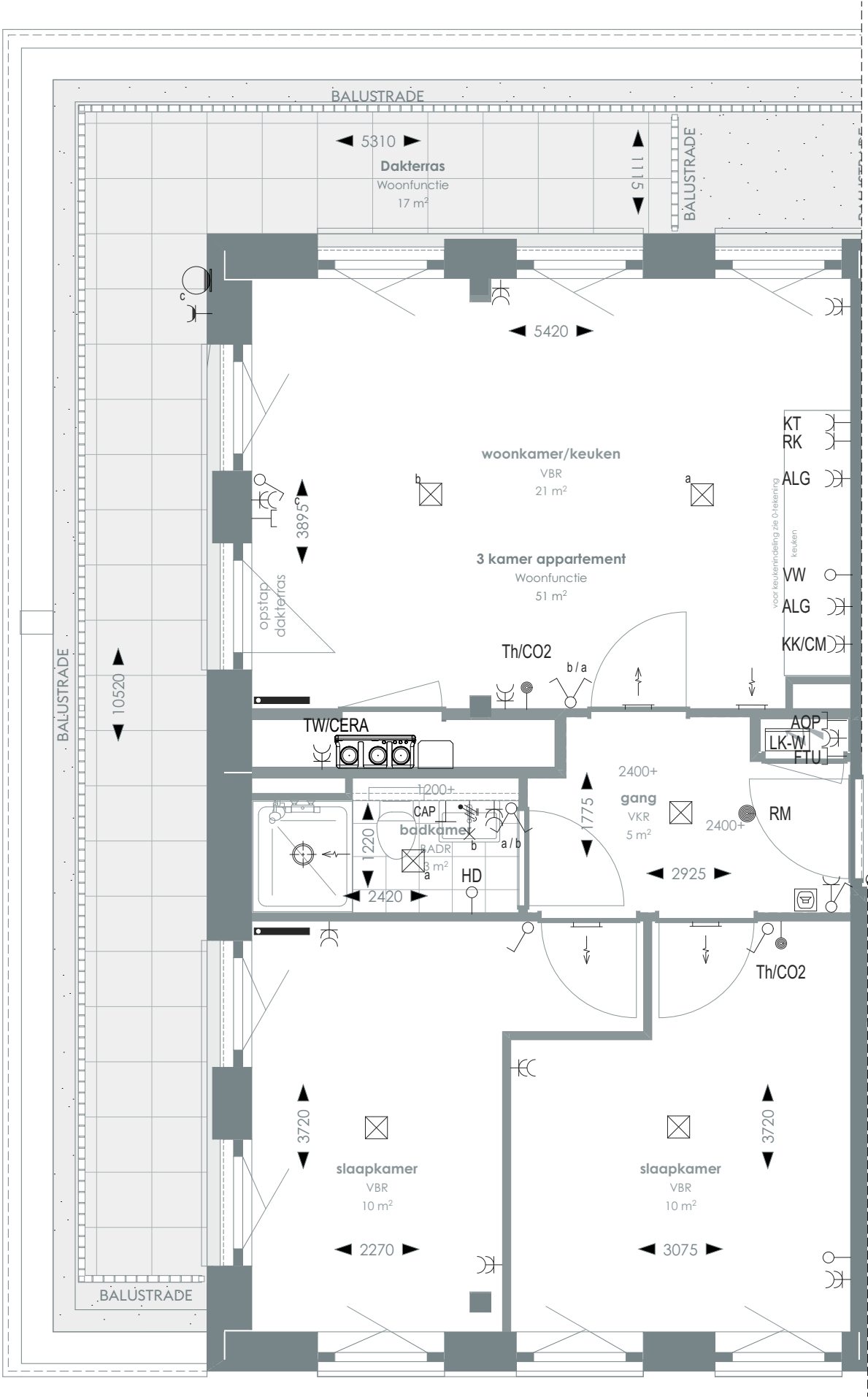
1:50 PLATTEGROND
