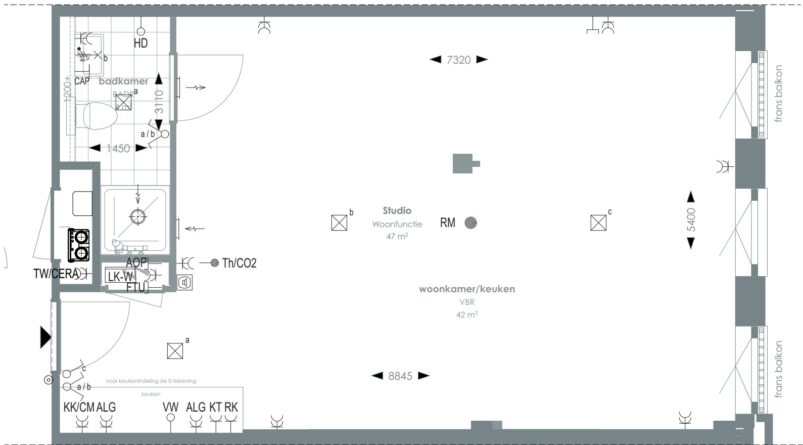
1:50 PLATTEGROND
