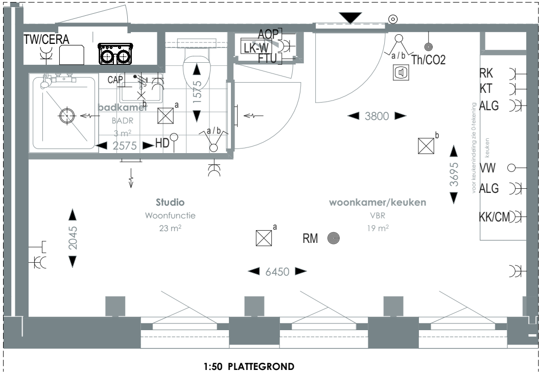
1:50 PLATTEGROND
