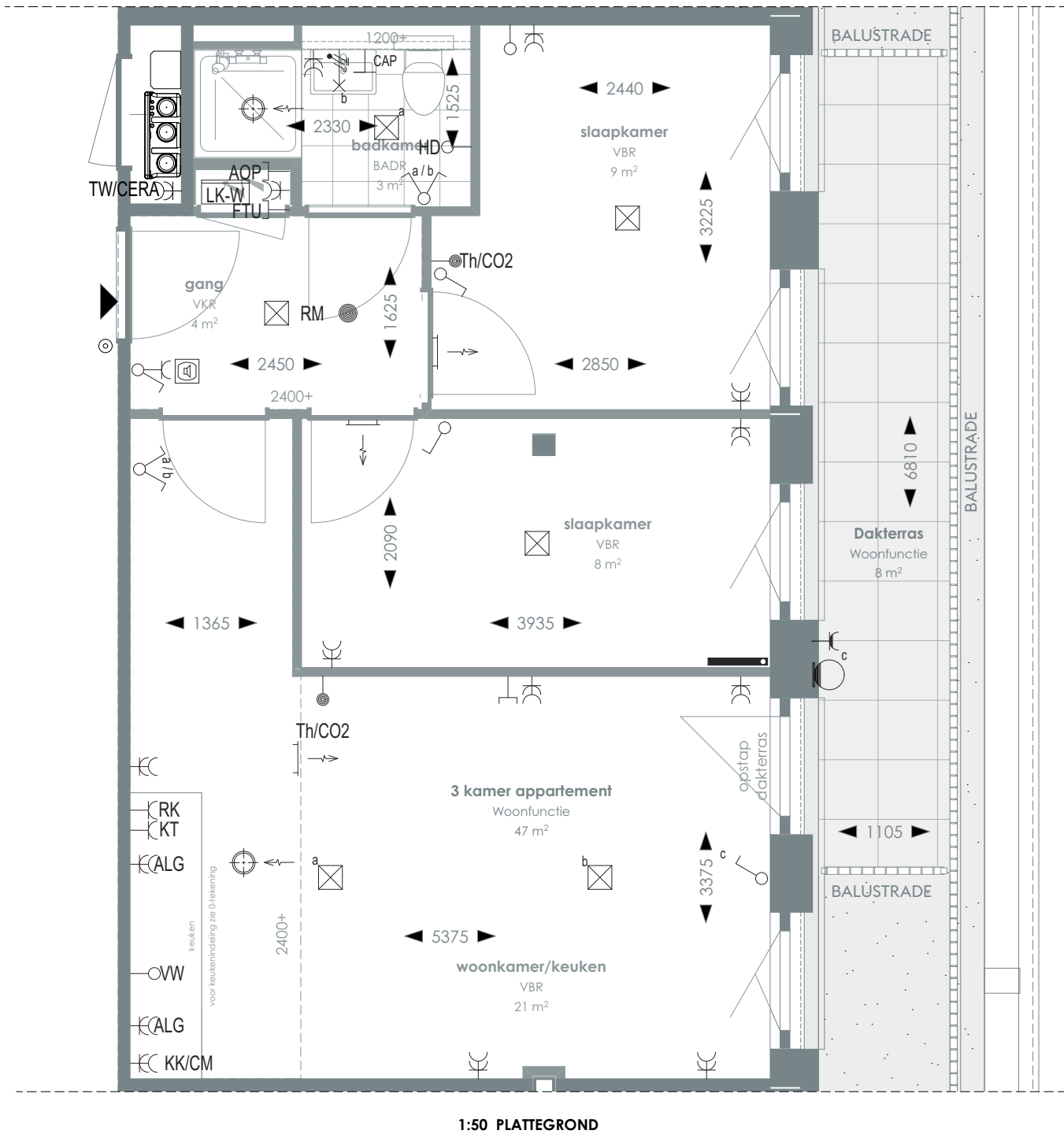
1:50 PLATTEGROND
