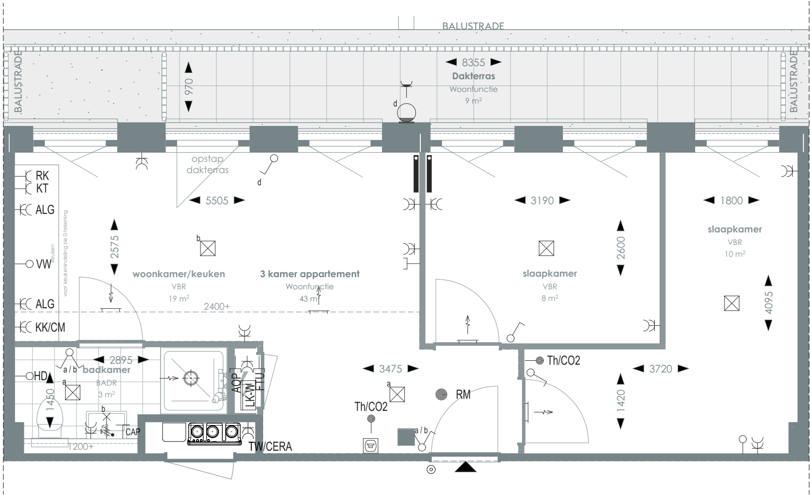
1:50 PLATTEGROND
