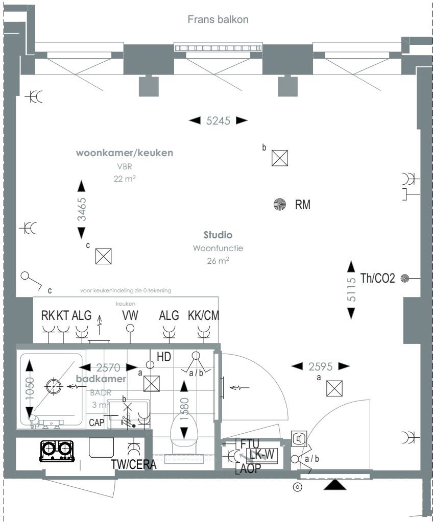
1:50 PLATTEGROND
