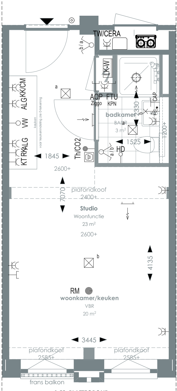
1:50 PLATTEGROND
