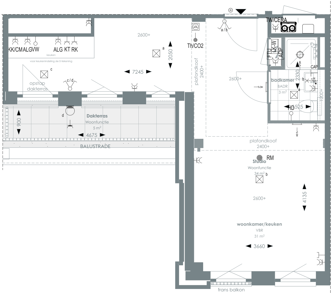
1:50 PLATTEGROND
