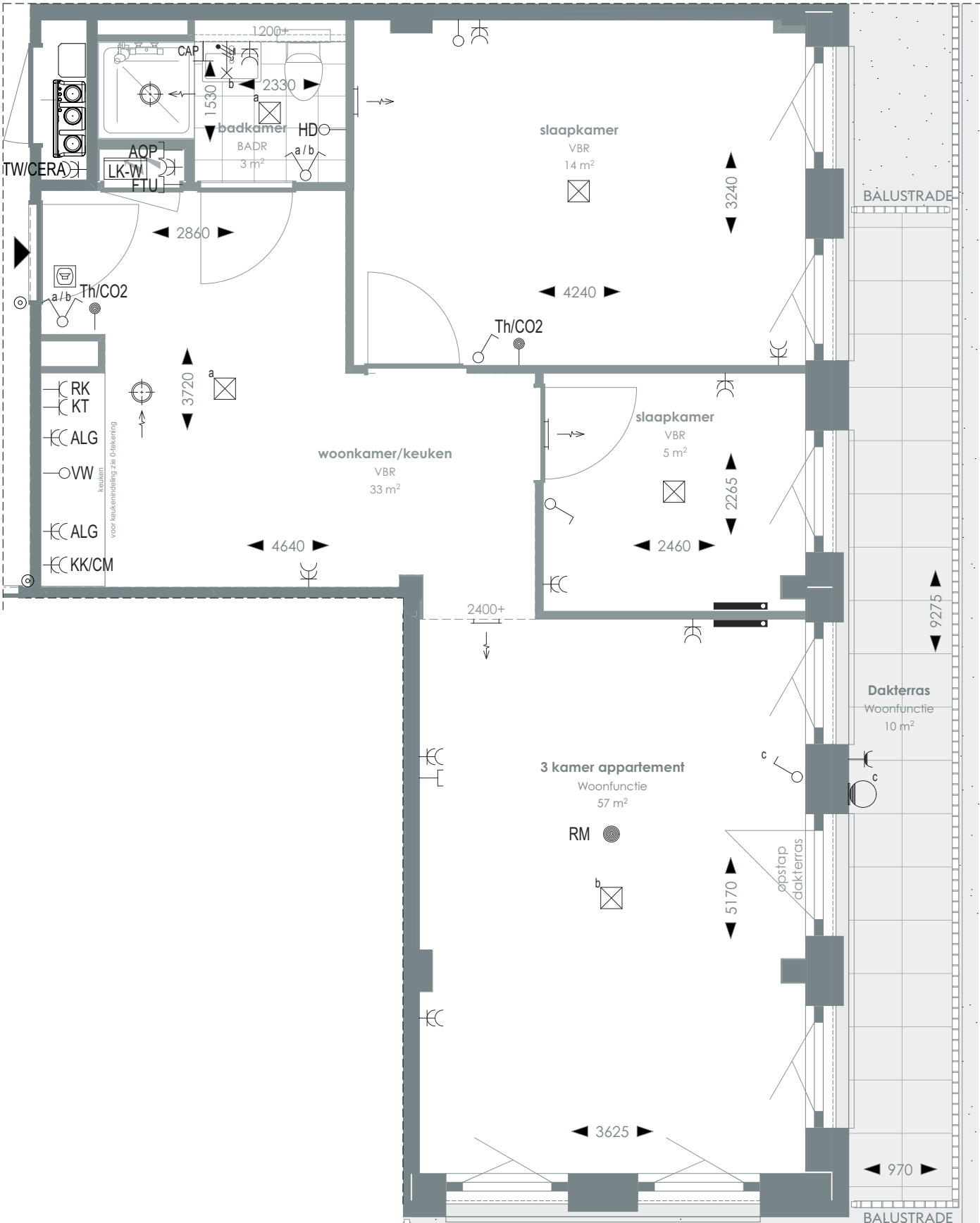
1:50 PLATTEGROND
