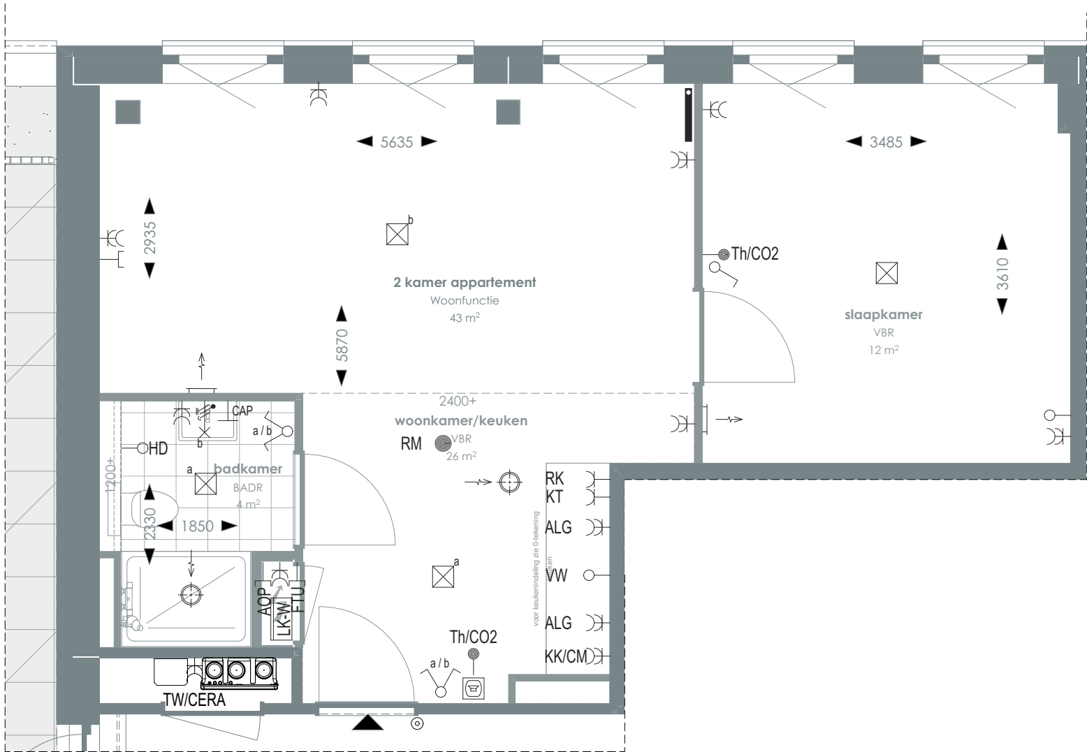
1:50 PLATTEGROND
