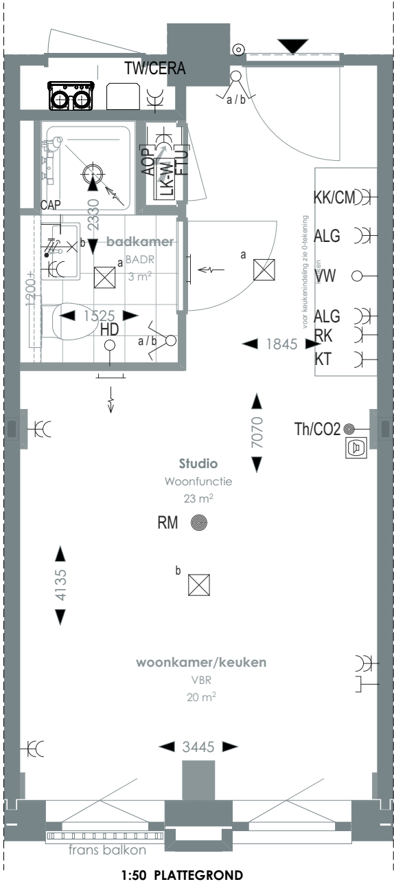
1:50 PLATTEGROND
