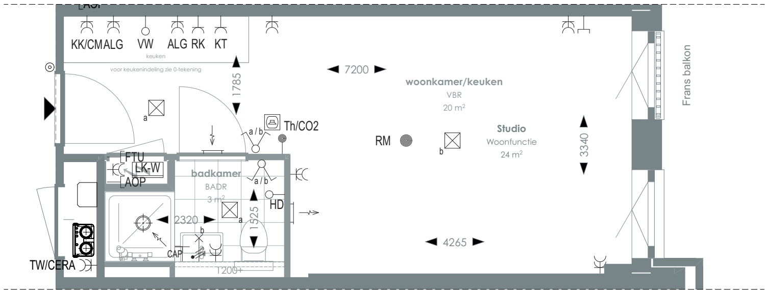
1:50 PLATTEGROND
