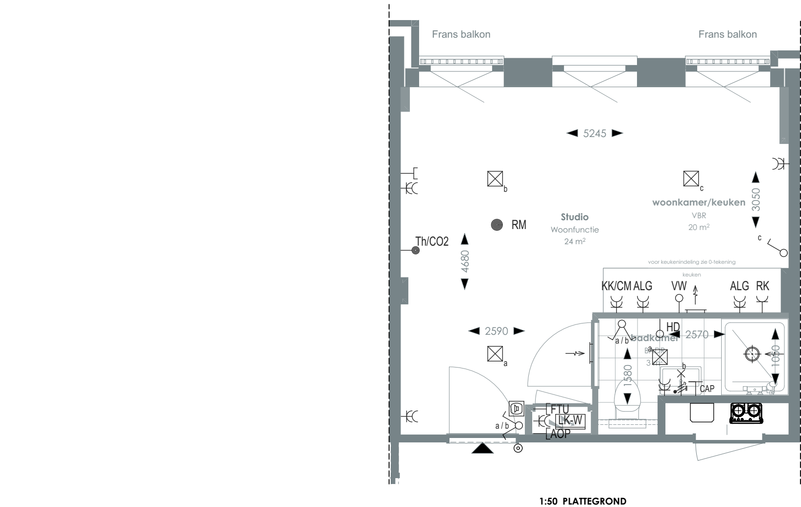
1:50 PLATTEGROND
