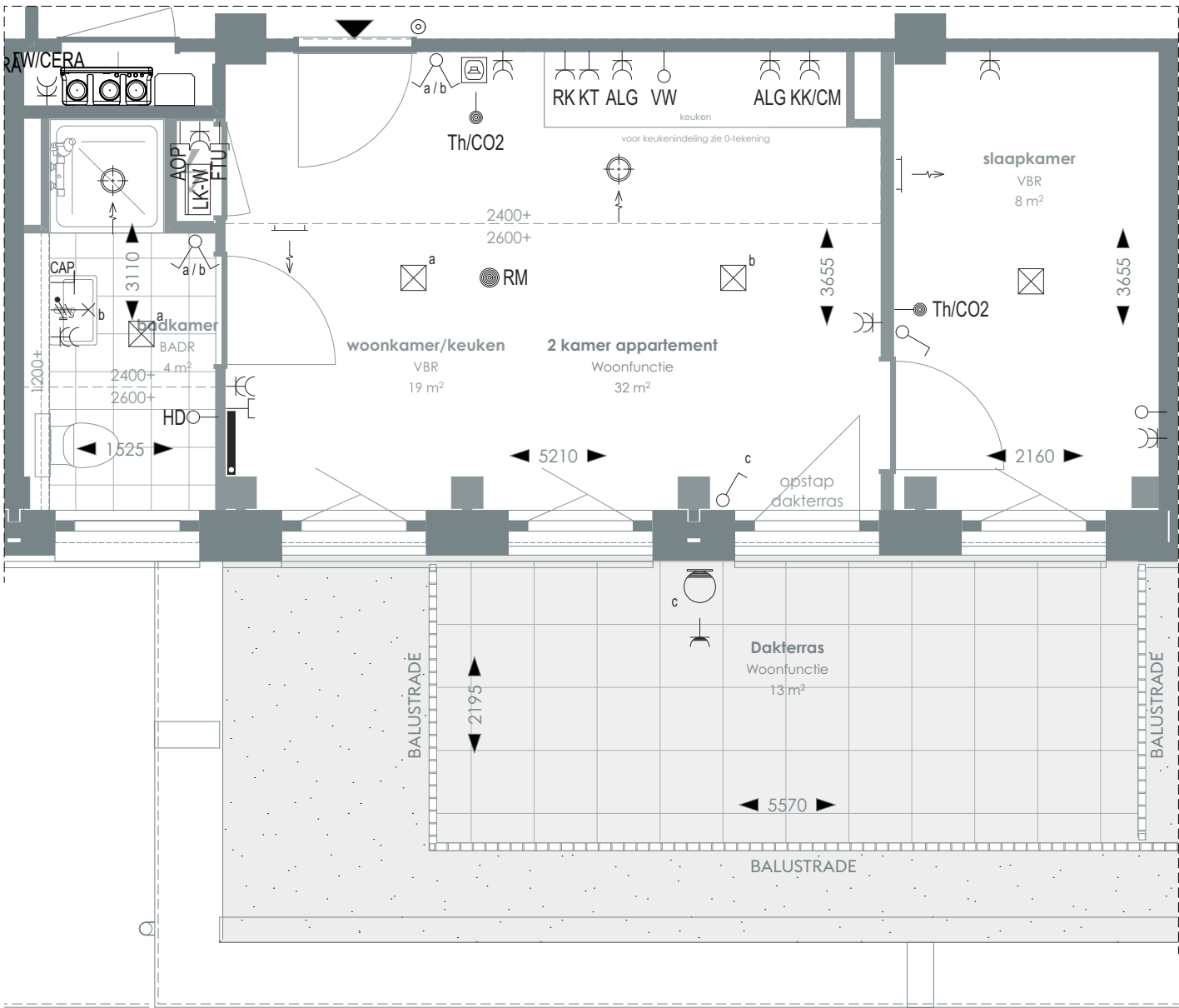
1:50 PLATTEGROND
