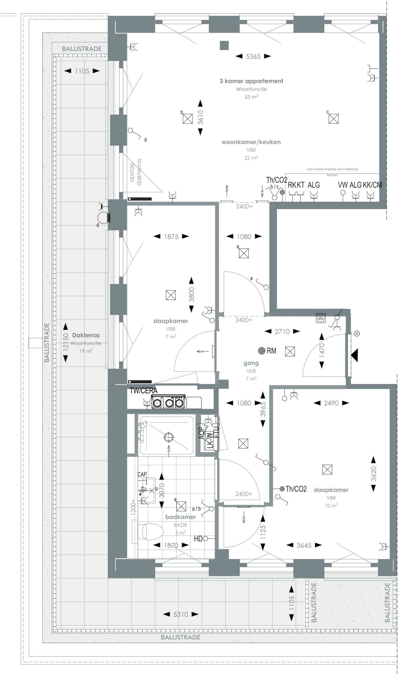
1:50 PLATTEGROND
