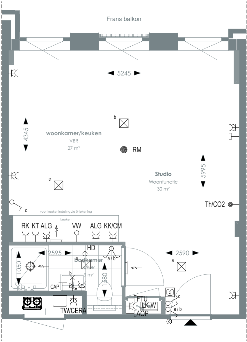
1:50 PLATTEGROND
