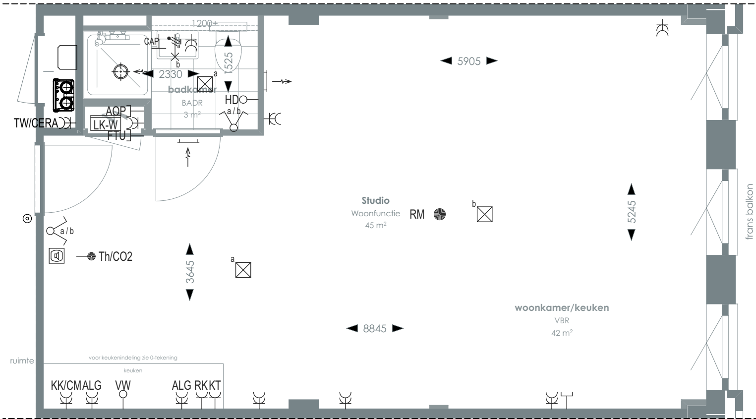
1:50 PLATTEGROND
