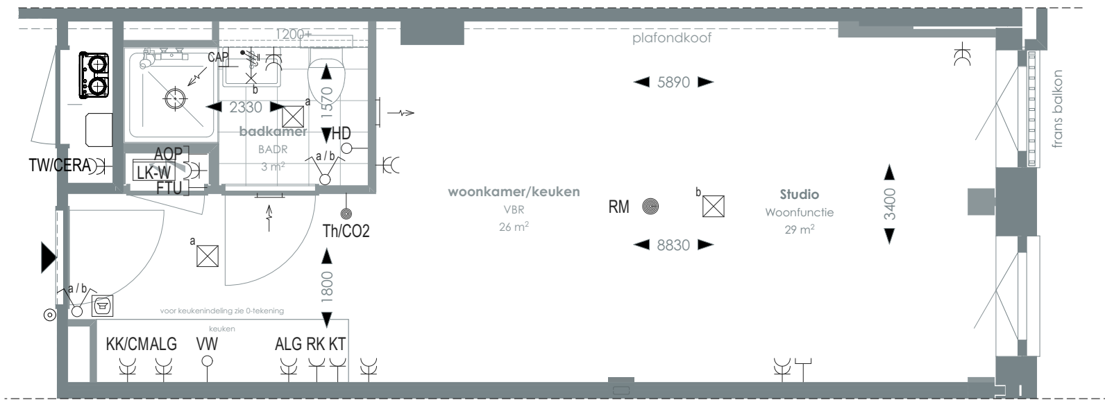
1:50 PLATTEGROND
