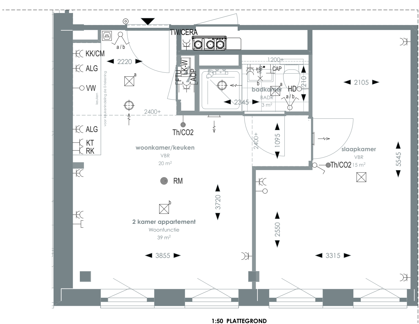
1:50 PLATTEGROND
