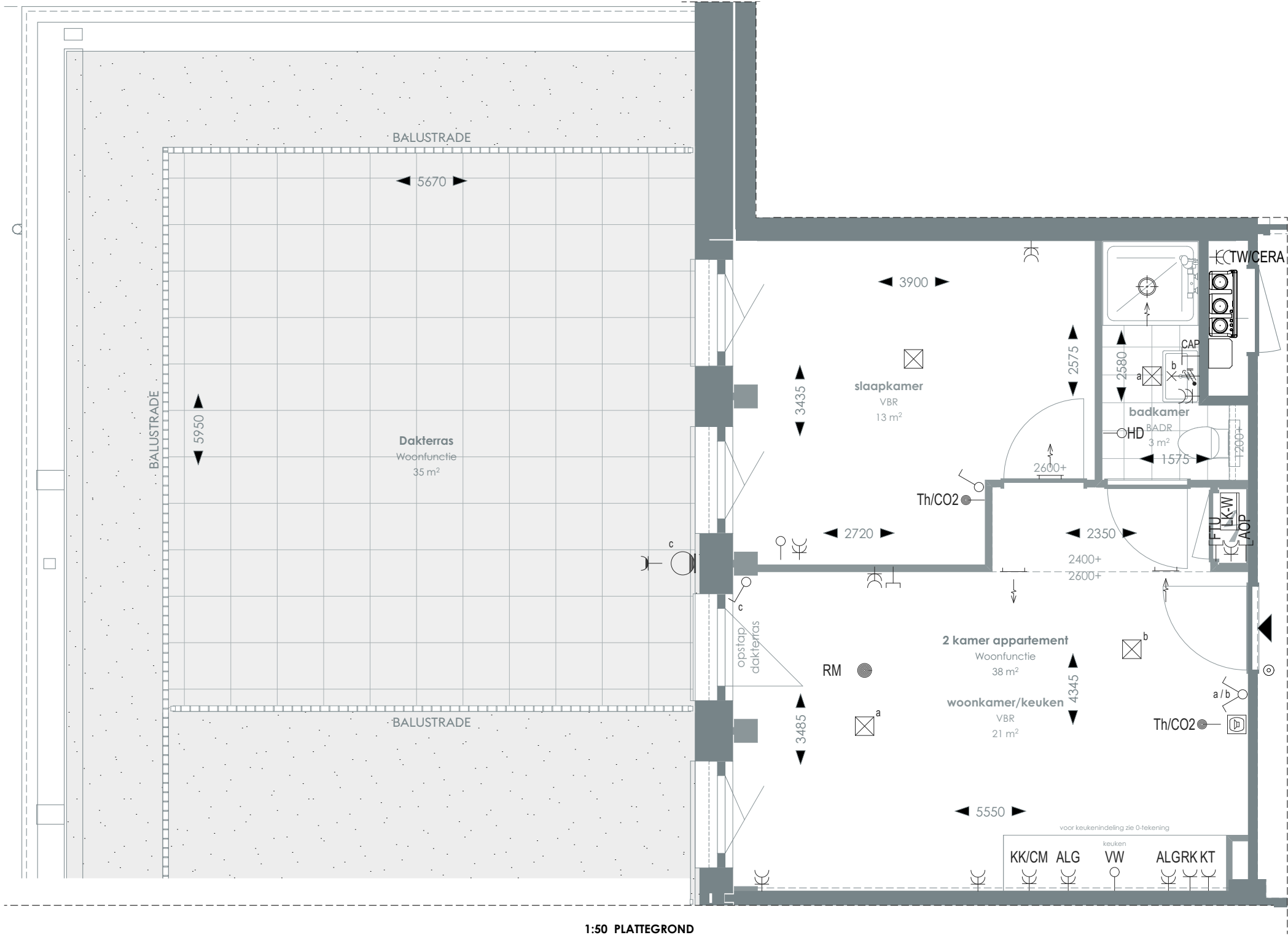
1:50 PLATTEGROND
