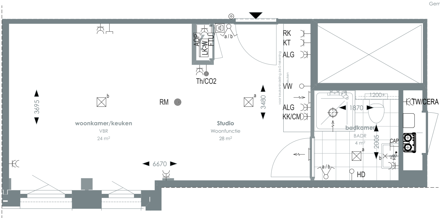
1:50 PLATTEGROND
