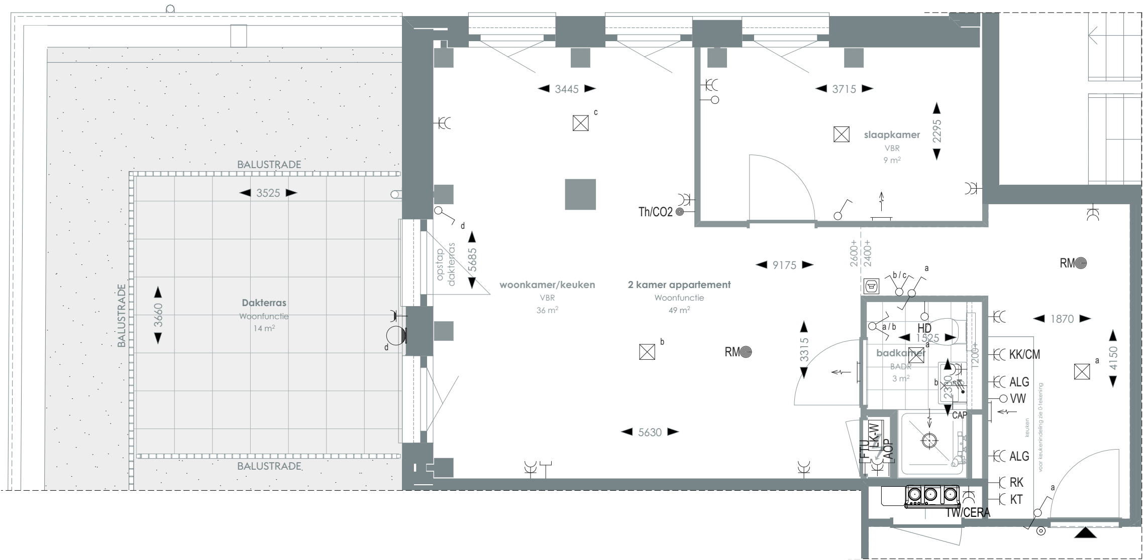
1:50 PLATTEGROND
