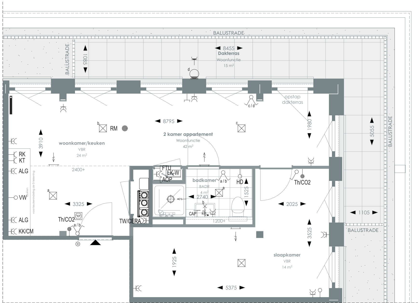
1:50 PLATTEGROND
