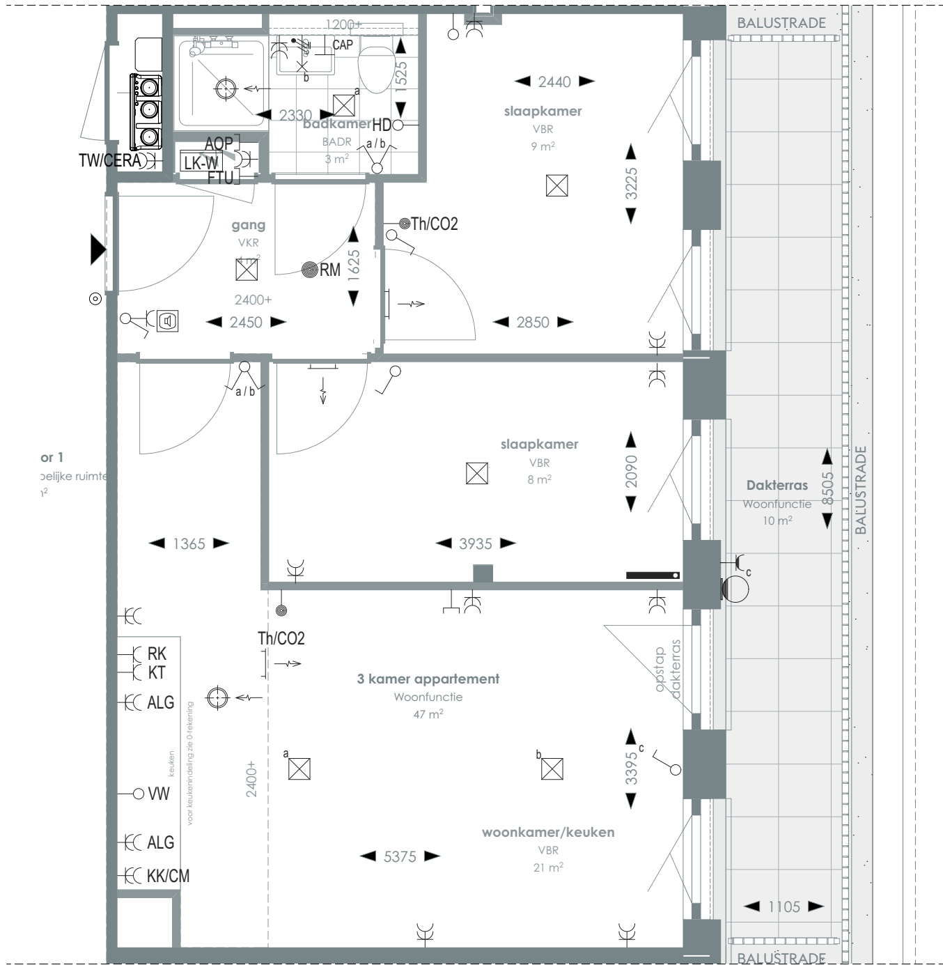
1:50 PLATTEGROND
