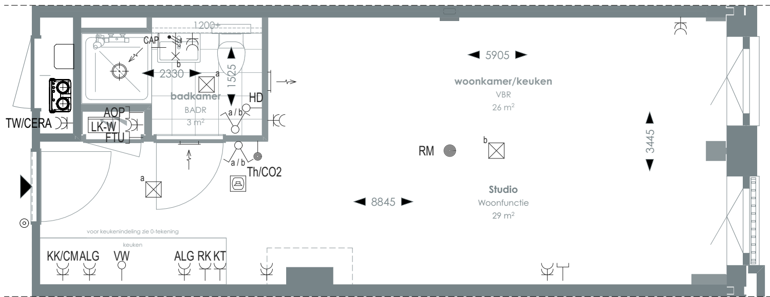
1:50 PLATTEGROND
