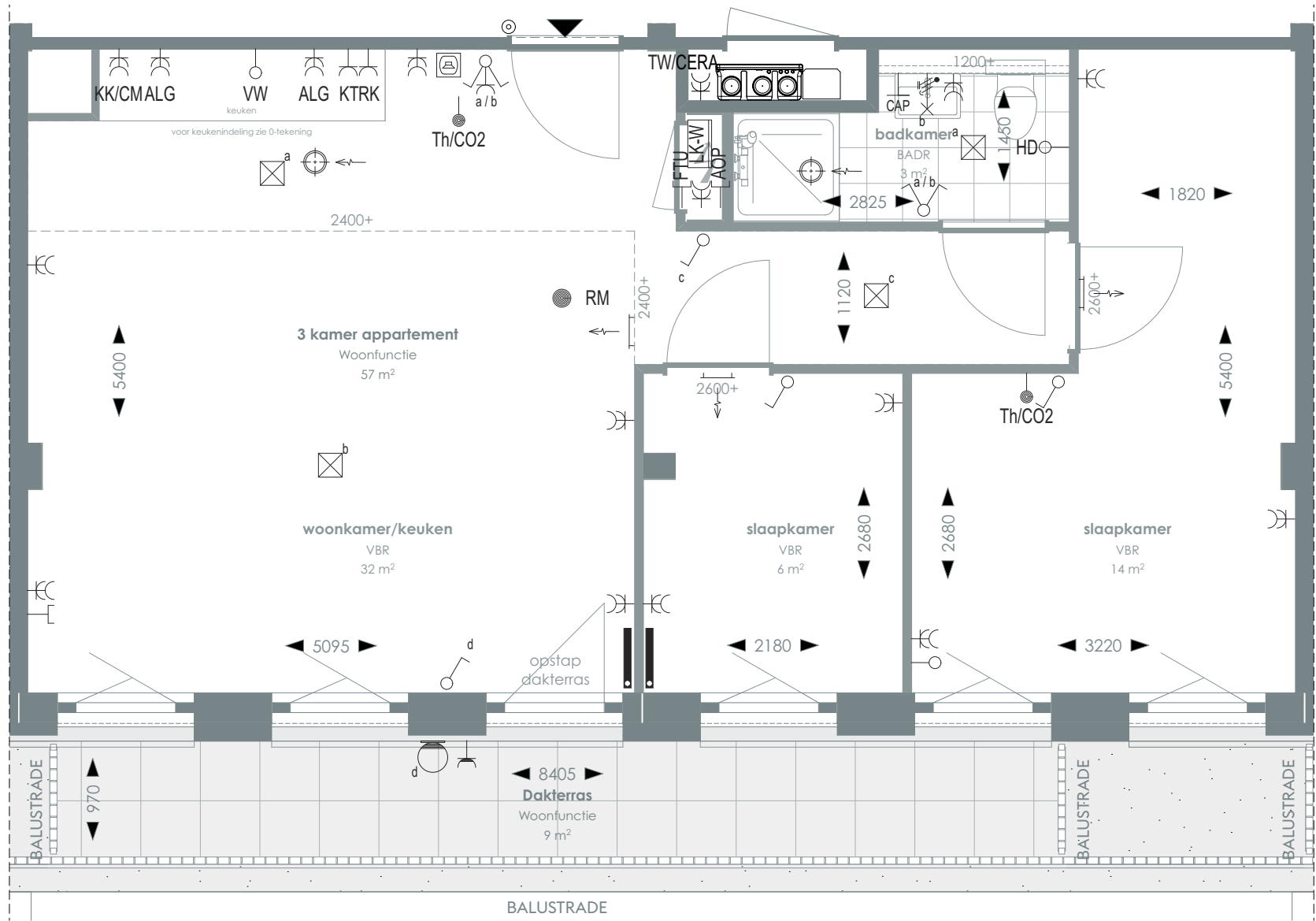
1:50 PLATTEGROND
