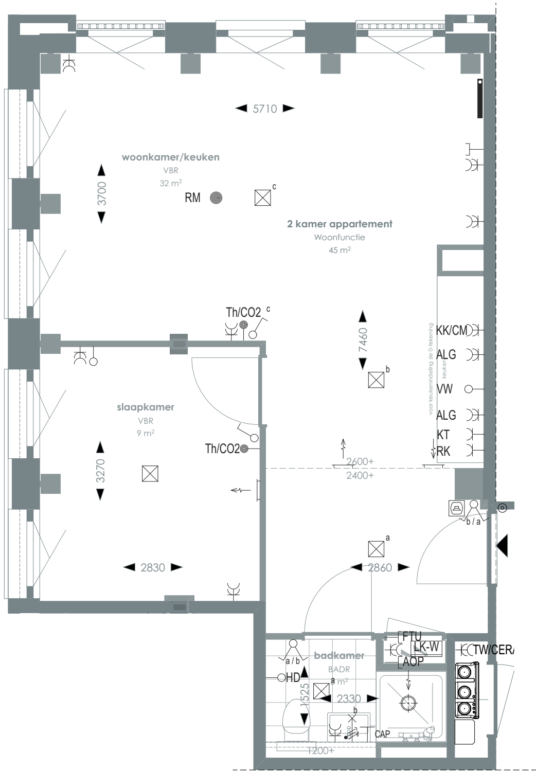
1:50 PLATTEGROND
