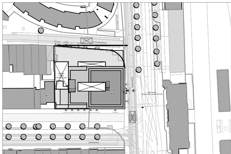
1:2000 SITUATIE
